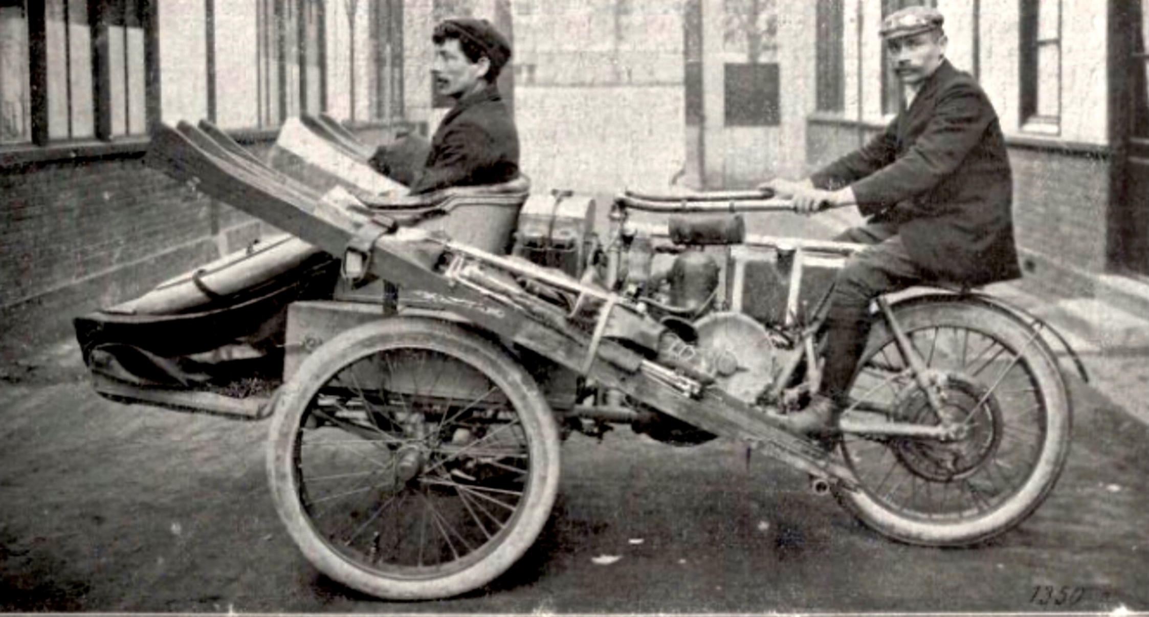
Fig. 1. — PÉRIN-PARIS. — Le mototri Contal en ordre de marche.
