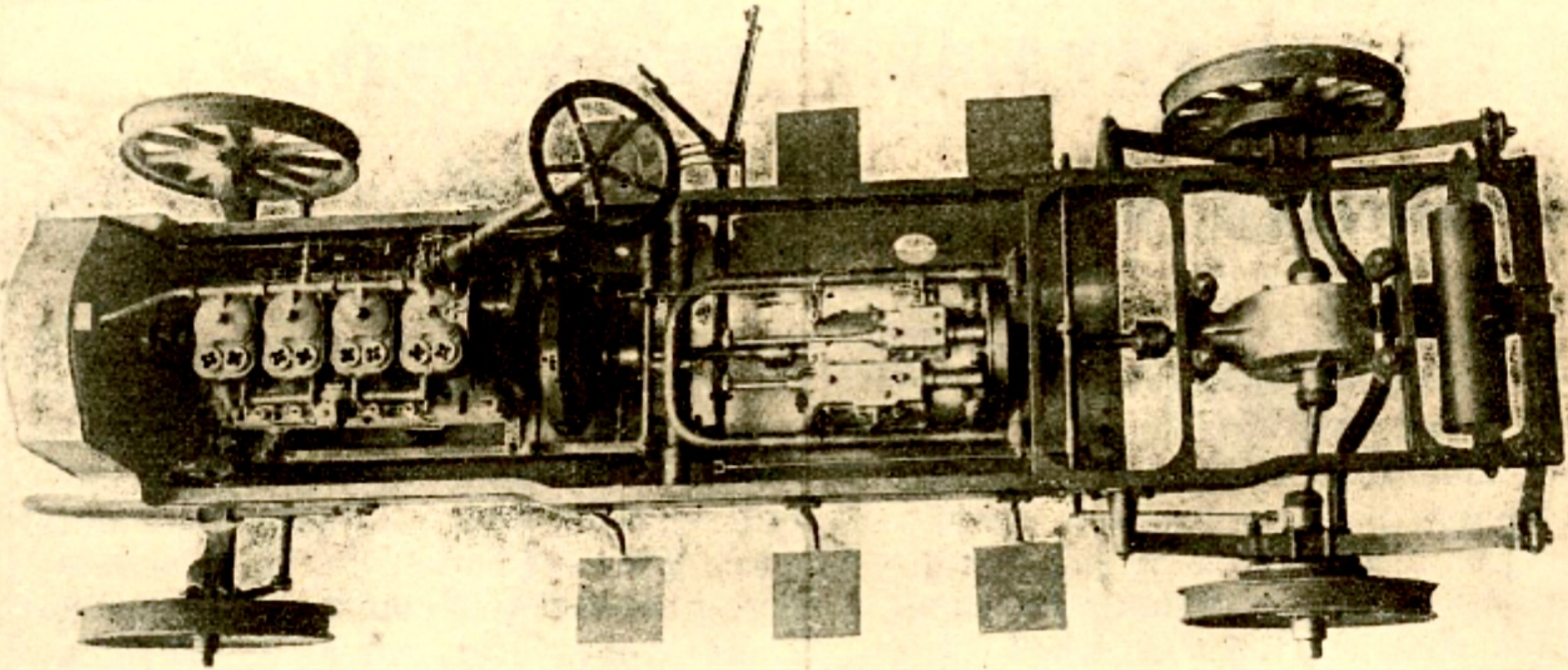
CHASSIS 30 CHEVAUX DE DION-BOUTON MODÈLE 1908 TYPE B J
