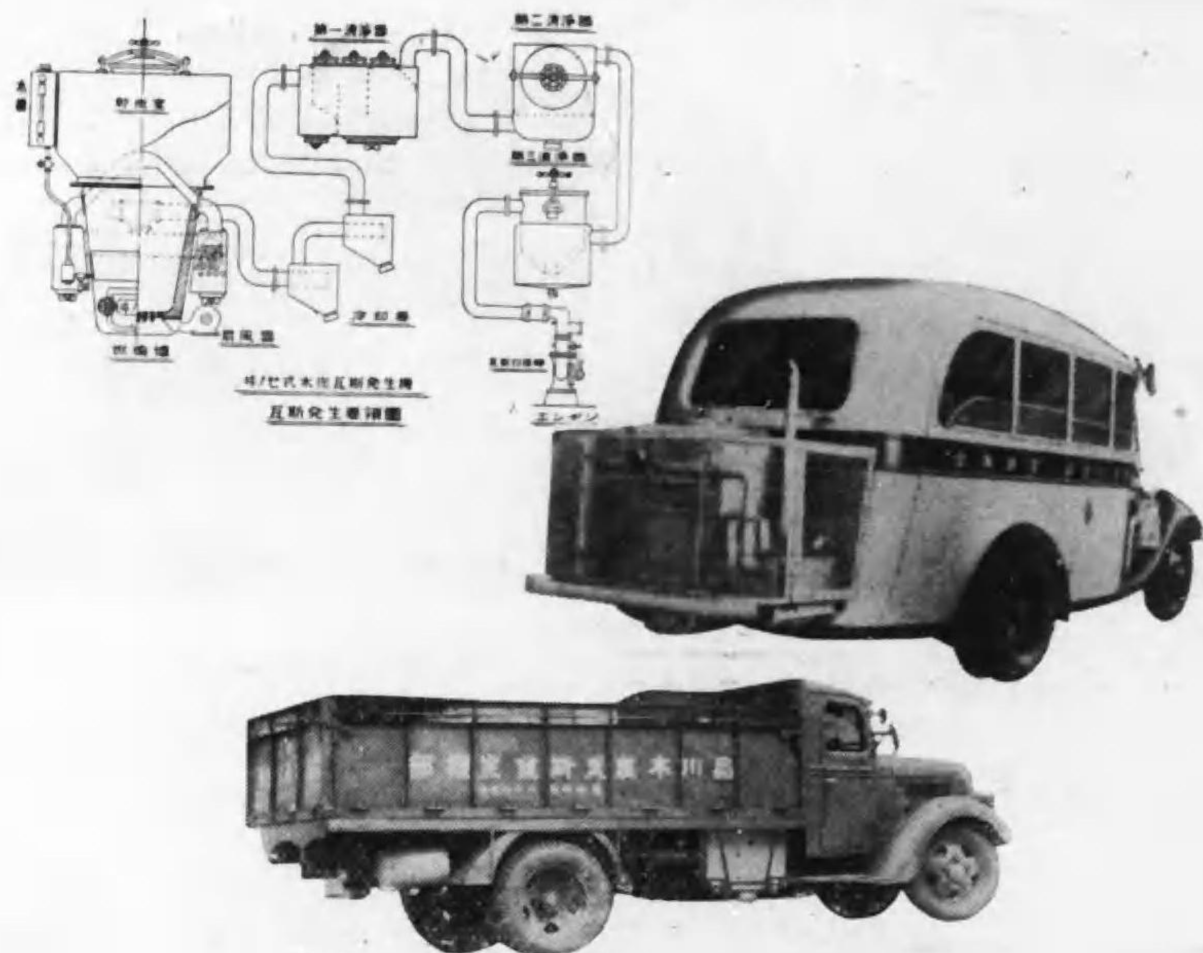
キノセ式木炭瓦斯発生機の概要
