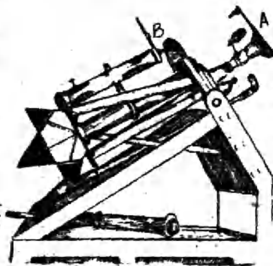
攝取星光彩色帶的裝置：星光由A處射入。經過三回三稜鏡。到B處，感影照像軟片上。C處是察測焦點的小孔。
