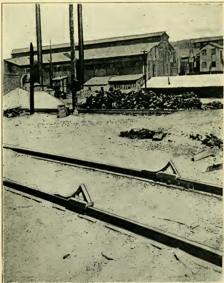
FIG. 8.—“SABOT FRIEN” BRAKE SKID.
