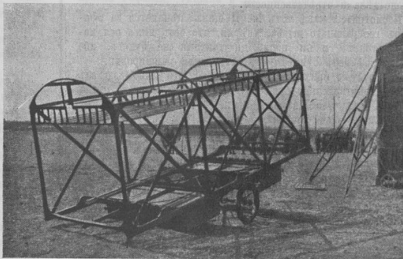
Катки для перевозки двуплановъ на французскихъ маневрахъ.
