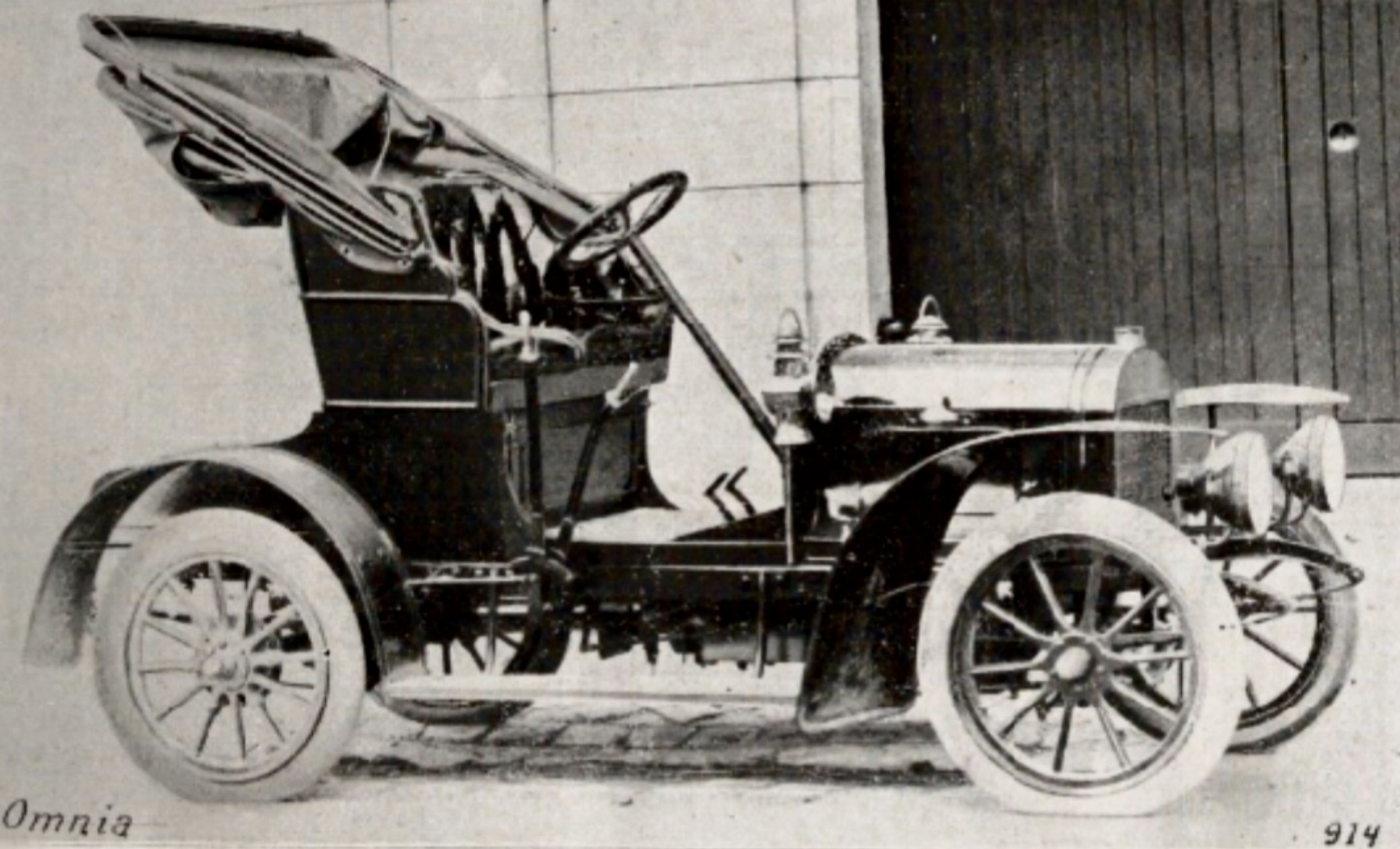
Fig. 1: — La voiturette Doriot, Flandria et C e .
