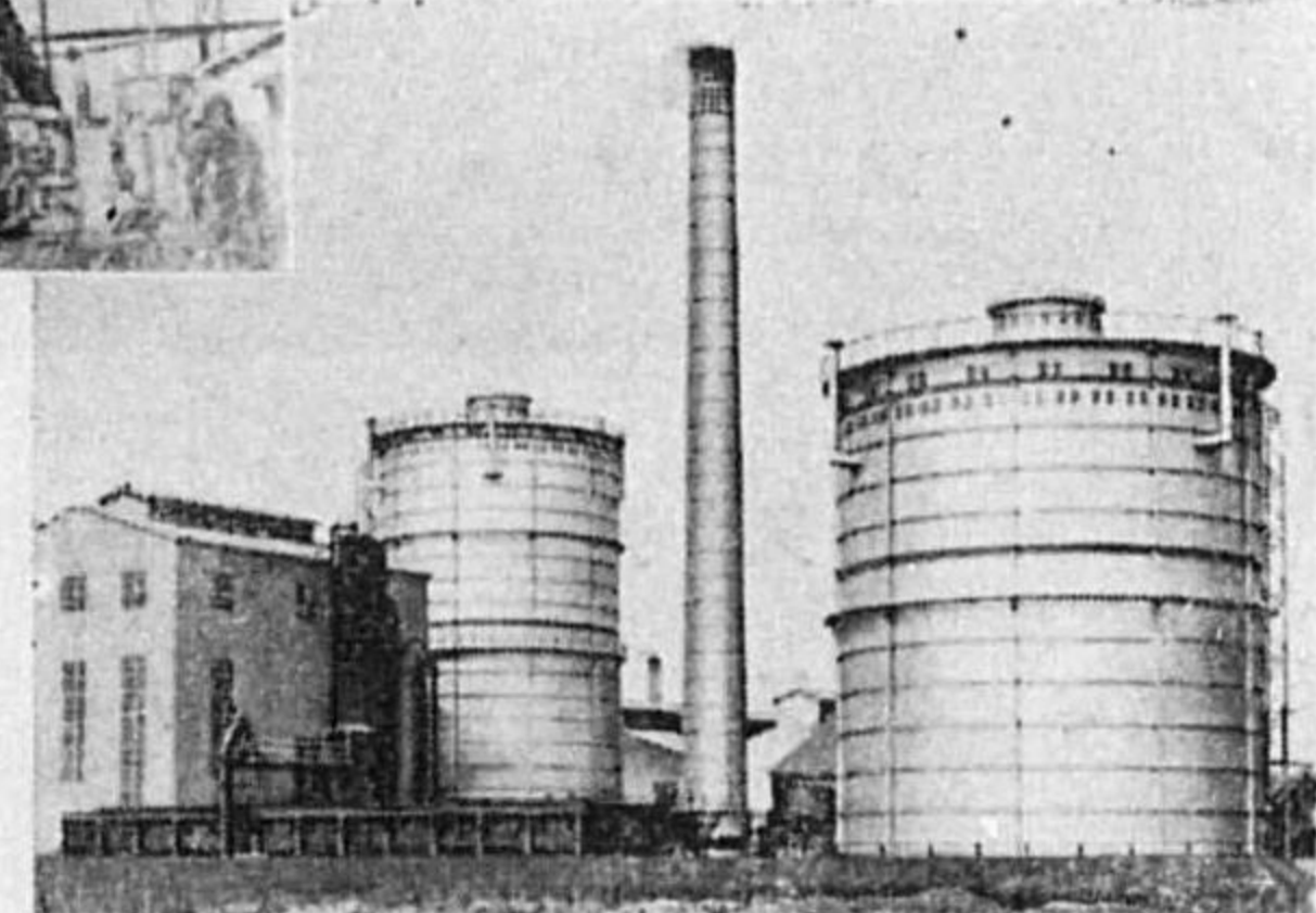
同上 5,000 立方米並 3,000 立方米 無水式瓦斯館
