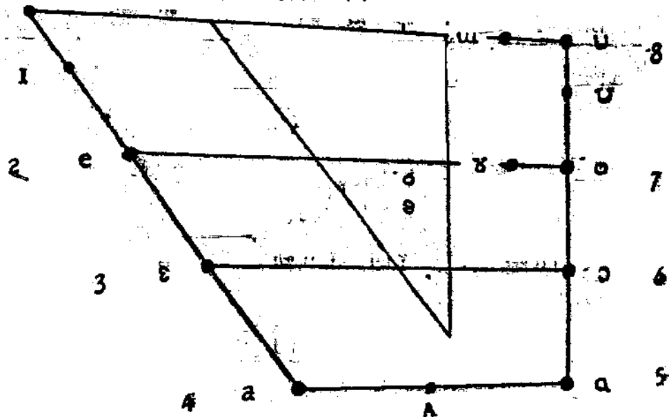
潮音元音發音舌位圖
