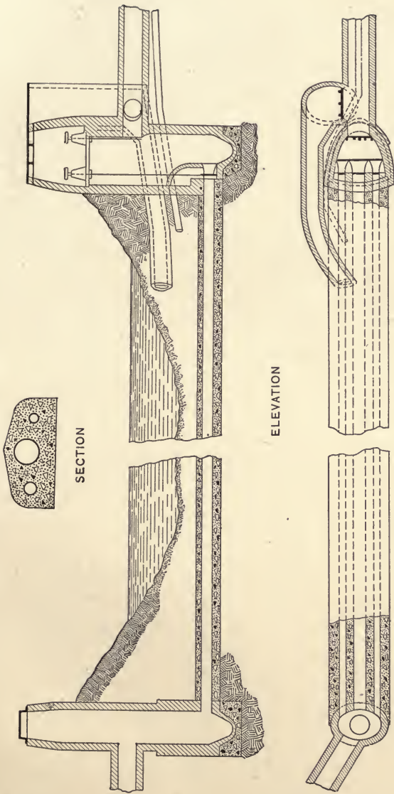
PLAN Fig. 118
