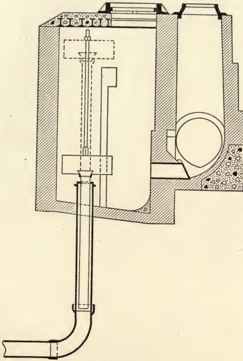
ELEVATION
