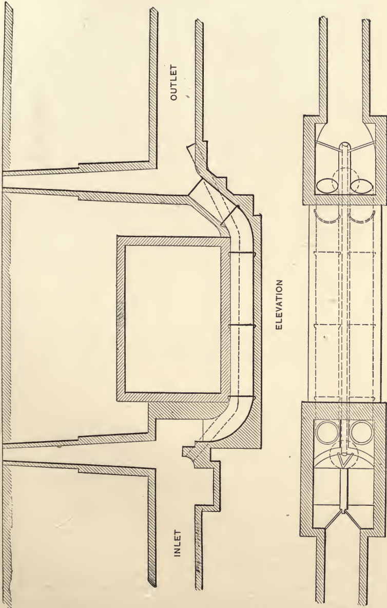
PLAN Fig. 120
