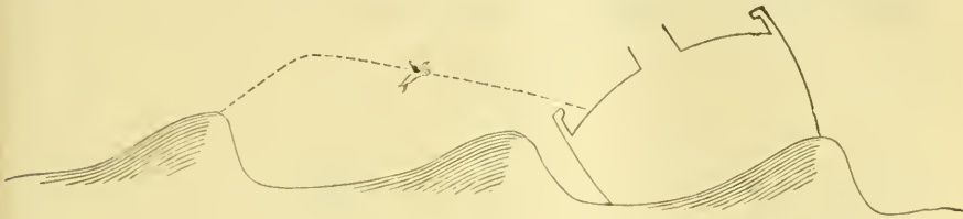
Flugbahn eines fliegenden Fisches, der auf Deck eines Schiffes niederfällt.
