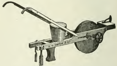
Fig. 200. A one-horse corn-planter.
