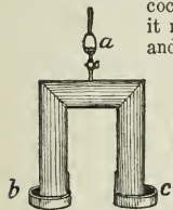
Fig. 657. A good siphon.
