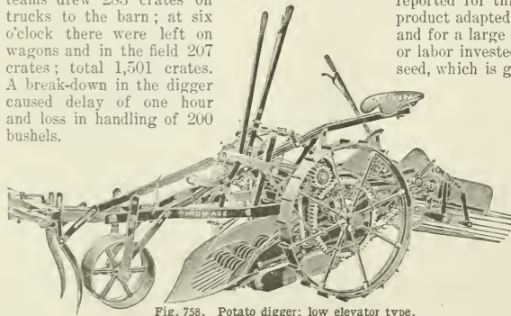
Fig. 758. Potato digger; low elevator type.
