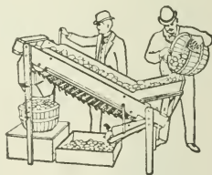
Fig. 760. Potato sorter.
