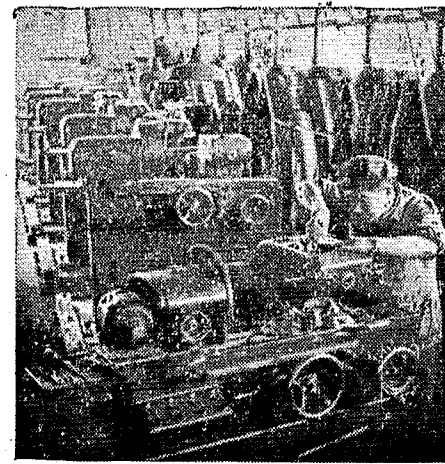
上海北江機器廠，在解放前能生產簡單機械，工人與工程師，在共同的努力下，已能製造出各種精密的機器，這正是我國工人正在裝配國內國產機器，這正是我國工人正在裝配國內國產機器的最偉大的成就。
