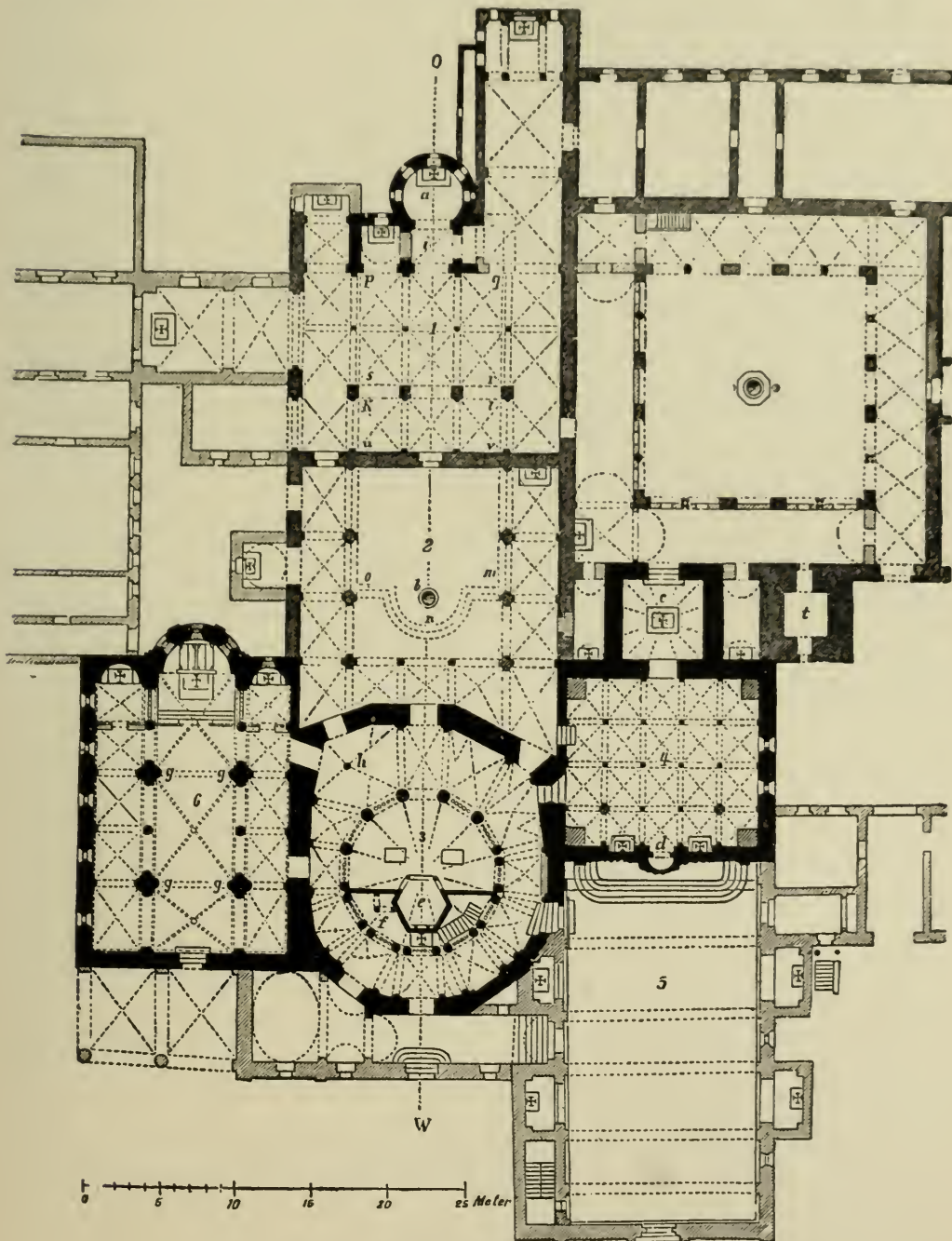
Fig. 67. Plan of S. Stefano, Bologna.
