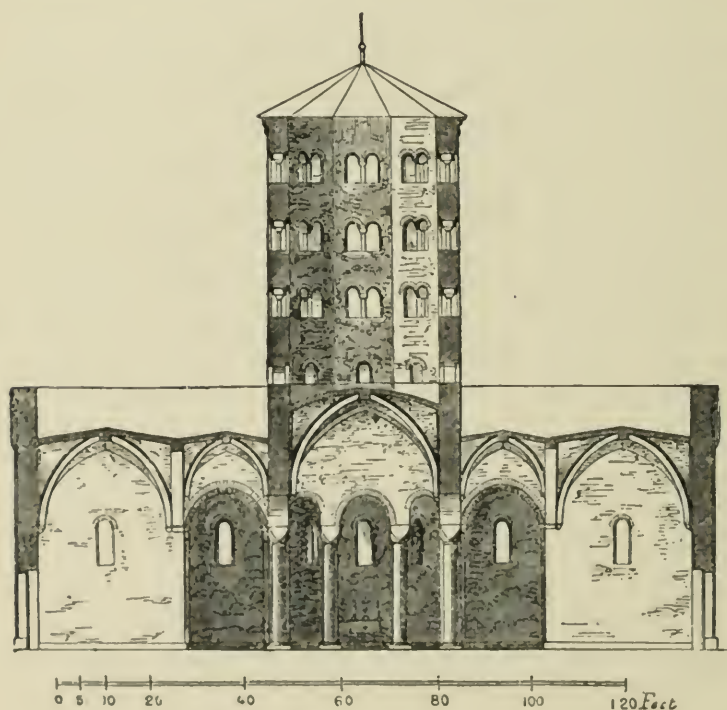
Fig. 72. Section, S. Antonino.
