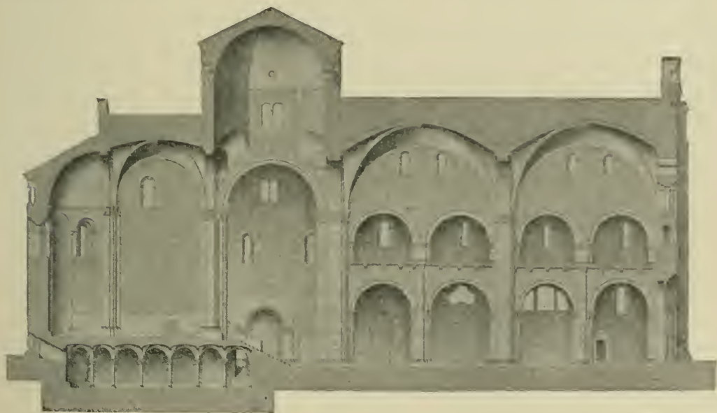
Fig. 65. Longitudinal Section of S. Michele.
