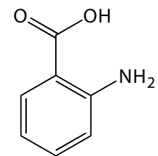
2-aminobenzoic acid
