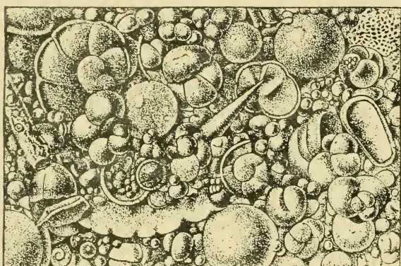
Globigerinenschlamm (nach Murray und Renard) 20 / 1 .
