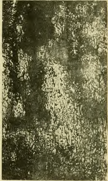
Faserstruktur des Meereises bei einem Schnitt senkrecht gegen die Oberfläche. Bei L Luftblasen. Die Kornstruktur ist aus dem helleren und dunkleren Schatten erkennbar.
