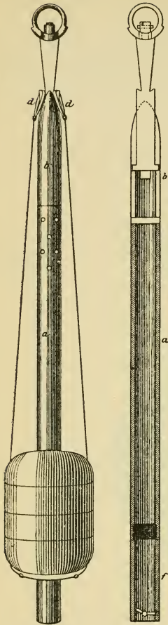
Das Hydra- oder Bailliolot.
