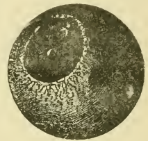
Schwarzes Meteor-eisenkügelchen, 20mal vergrößert (nach Renard)
