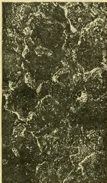
Kornstruktur des Gletschereises von einem Eisberge. Natürl. Größe. (Nach A. Hamberg.)
