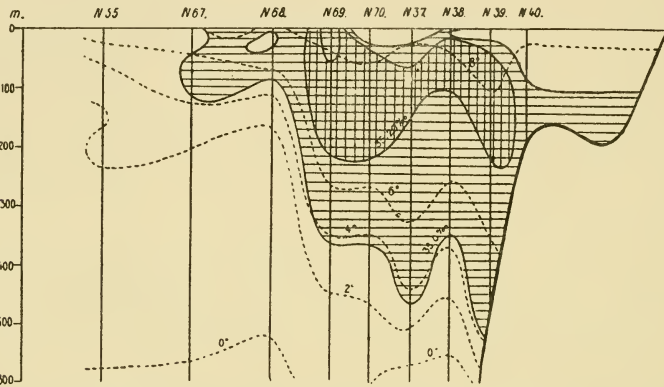
Temperatur- und Salzgehaltschichtung im norwegischen Meer westwärts von Kap Stadland im Mai 1904 (nach Helland-Hansen).
