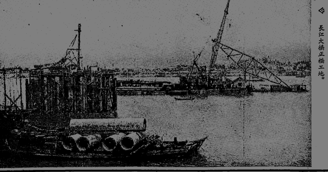
長江大橋正橋工程。
