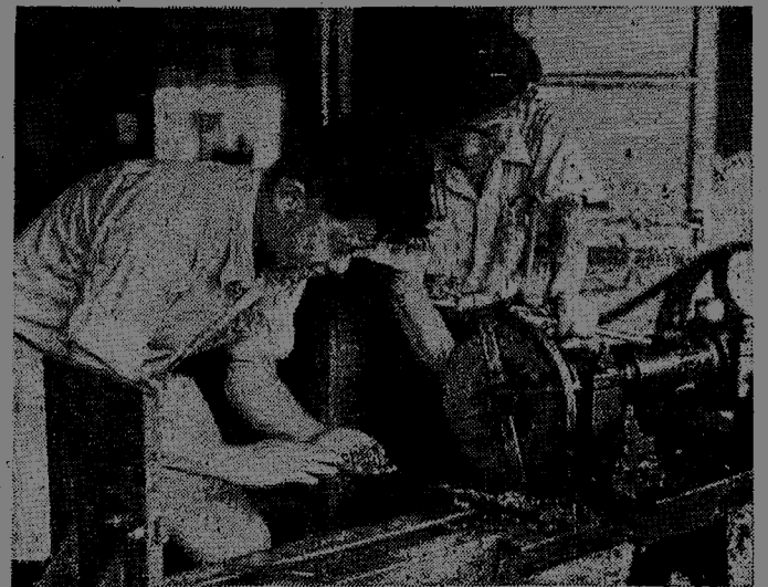
勘探隊附屬硯廠的老工人魯斌(右)和技術員李景錫改進了鋼粒切制機，保證了「鋼粒鑽進」法的順利推行。因為他們正在檢驗製出的鋼粒。
