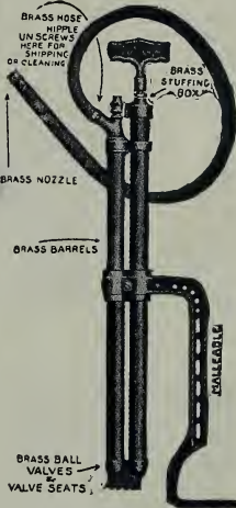
O. K. Bucket Pump
