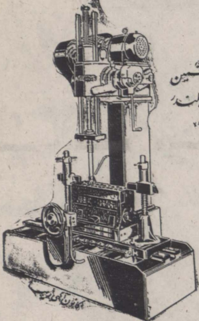
نماره ۵۹۰ ماشین تراش بزرگ کامپکت
