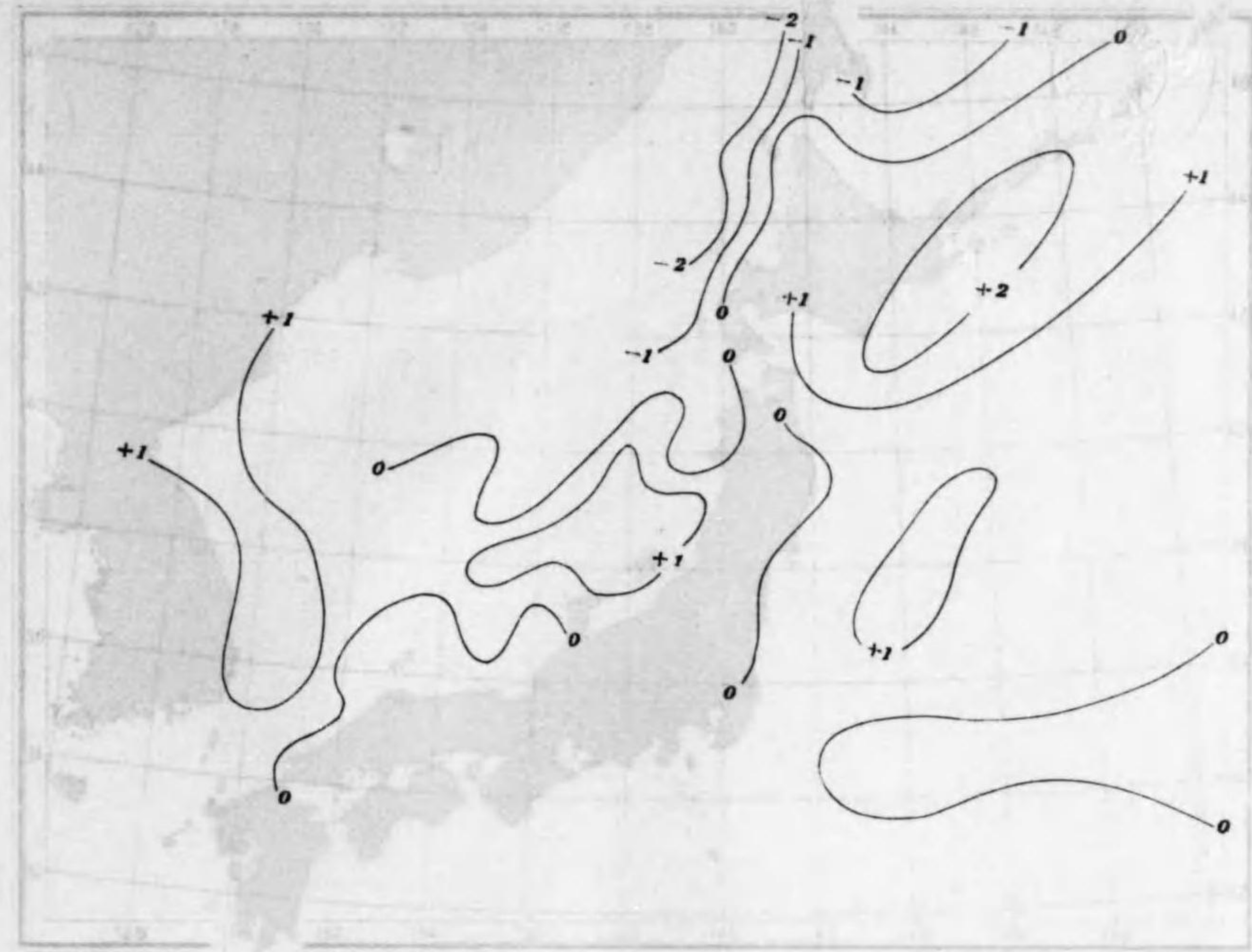
第四圖 本邦近海年平均氣溫偏差圖(攝氏)
