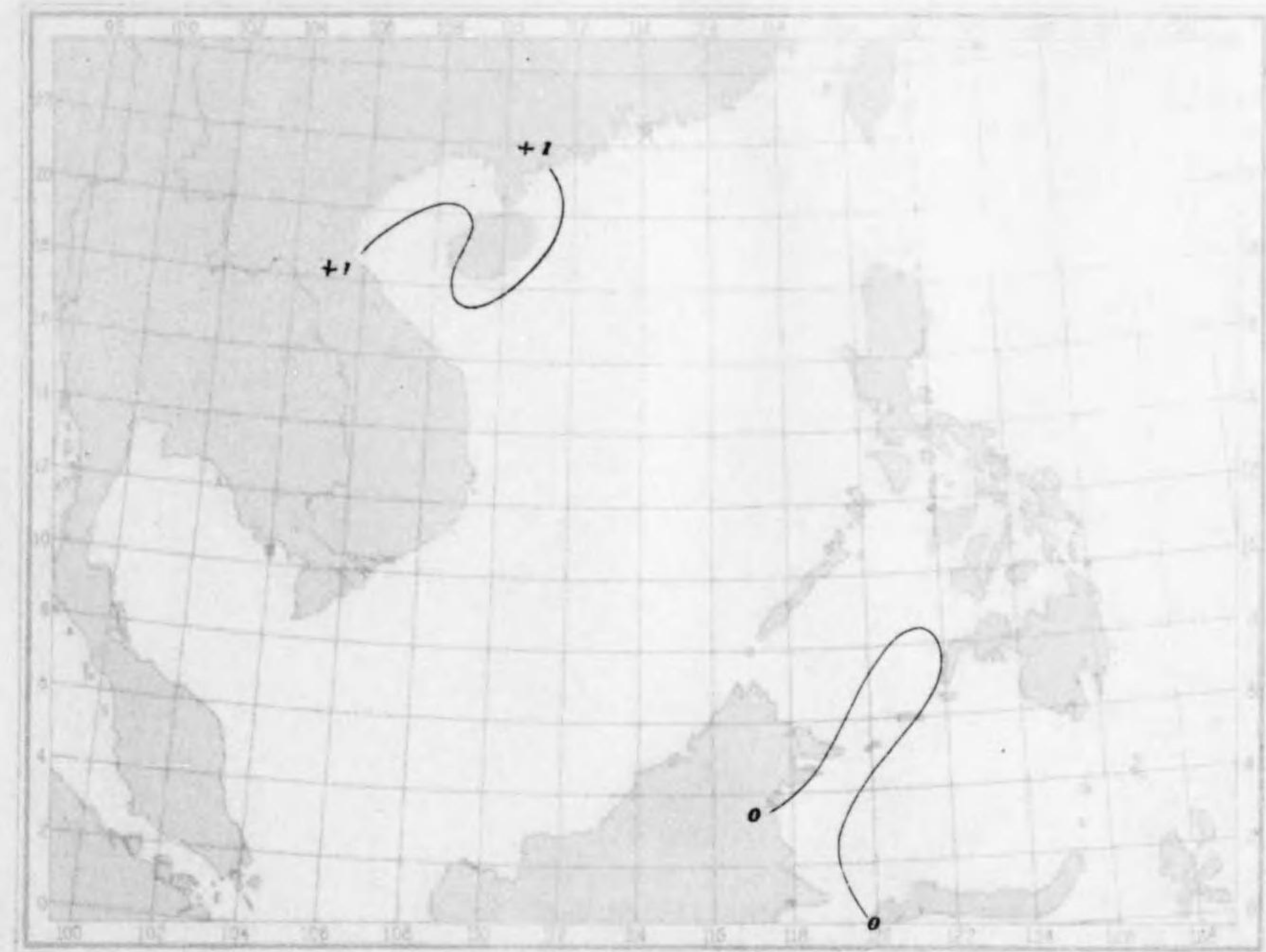
第九圖 南支那海年平均水溫偏差圖 (攝氏)
