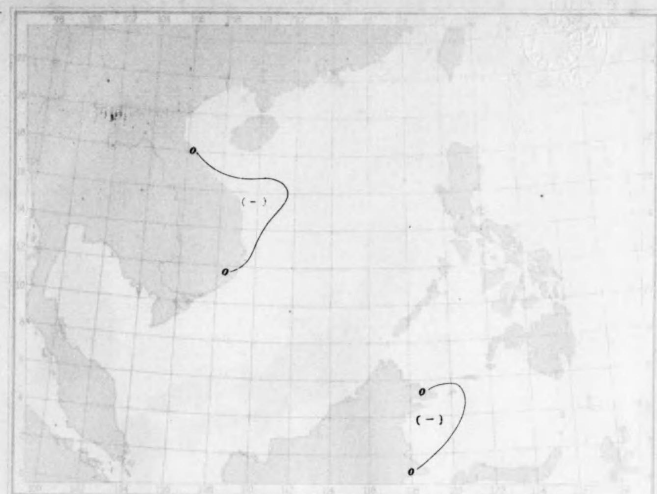
第八圖 南支那海年平均雨量偏差圖 (0-10)
