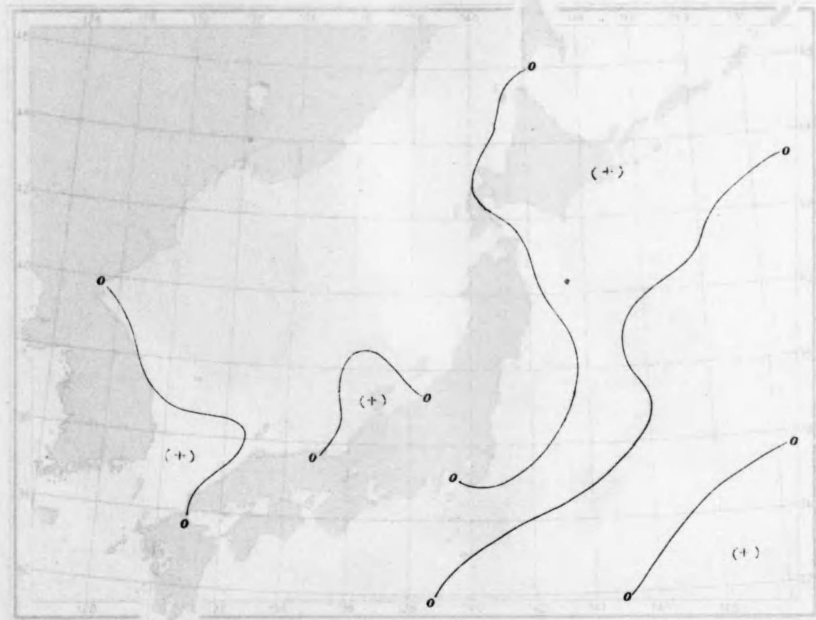
第五圖 本邦近海年平均雨量偏差圖(0-10)
