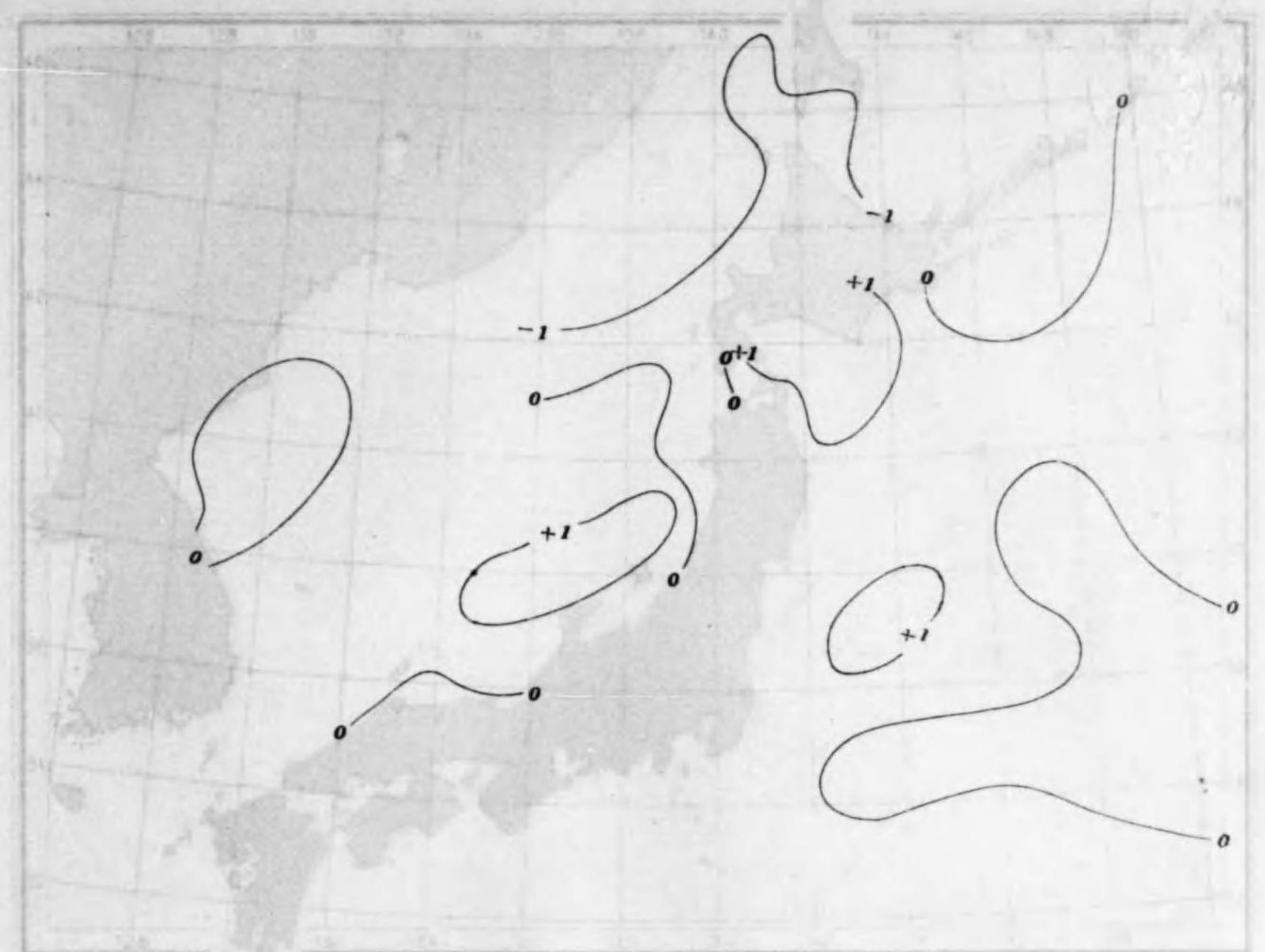
第六圖 本邦近海年平均水温偏差圖(攝氏)
