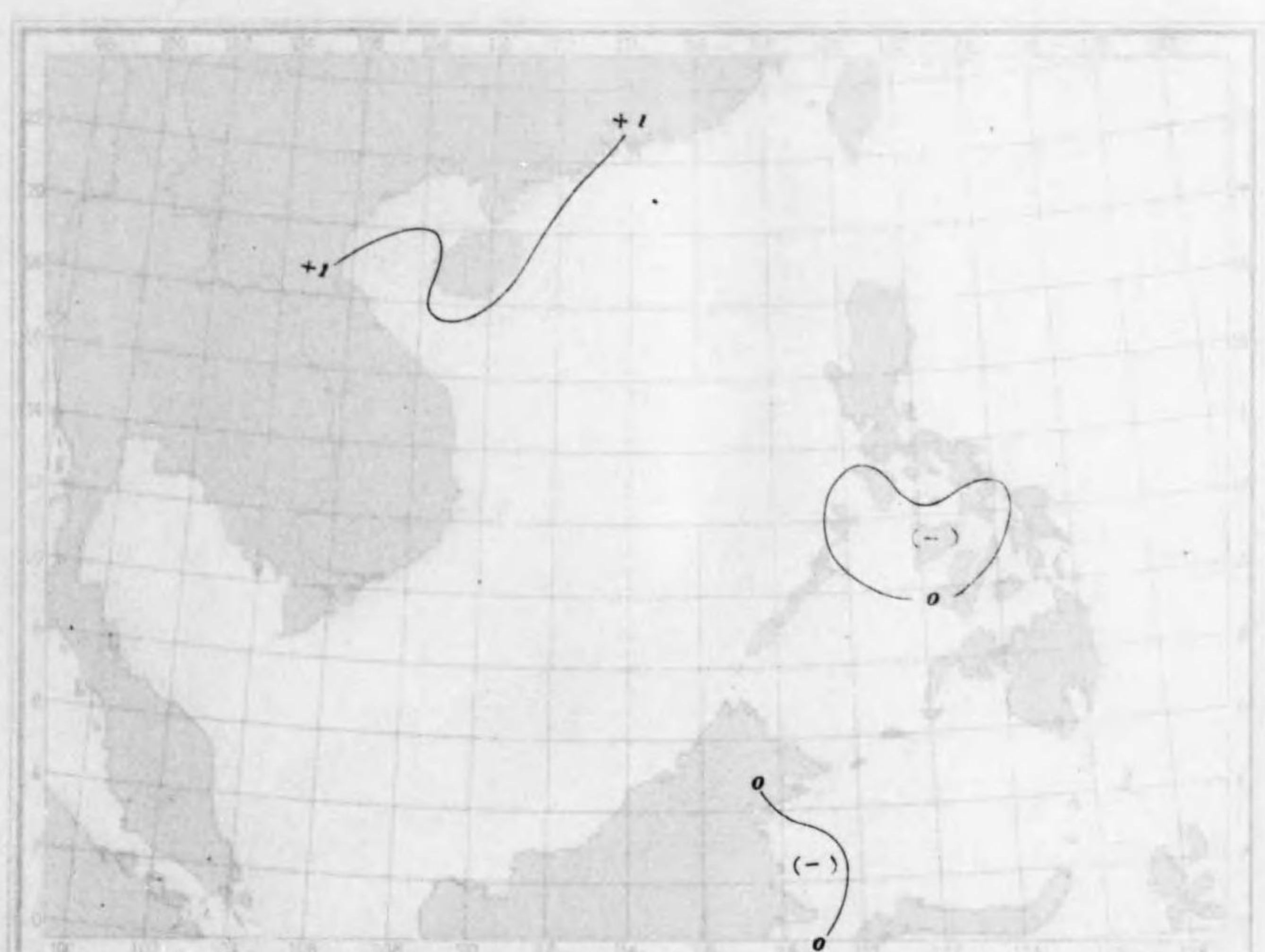
第七圖 南支那海年平均氣温偏差圖(攝氏)
