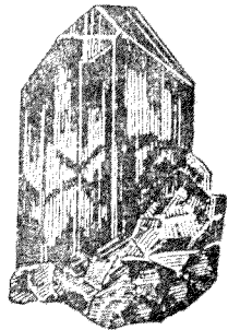
精黃
