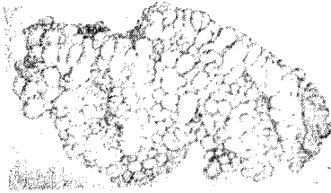
葡 萄 狀 石 髓
