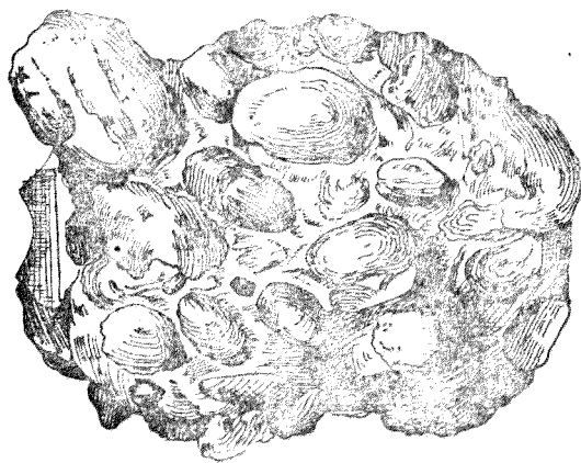
礫岩
