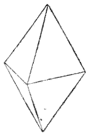
斜 錐 一
