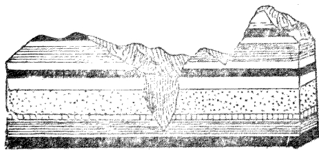
水之侵蝕谷
