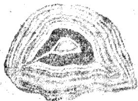
瑪 瑙
