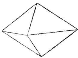
斜 方 錐
