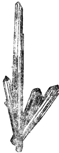
錫鑛
