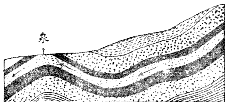
潛 水 及 湧 出 地 面 之 泉
