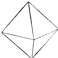
體面八
