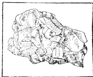
岩鹽之晶羣
