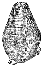
硫黃之結晶
