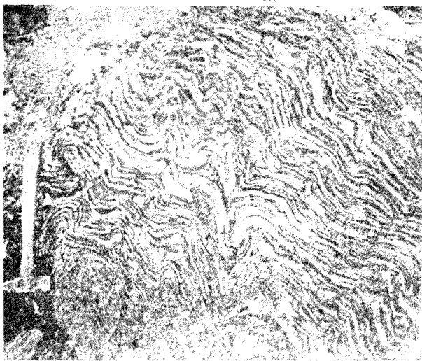
地層之褶曲
