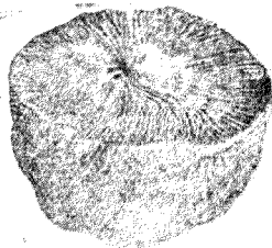
華化矽
