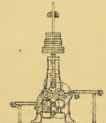
END ELEVATION
