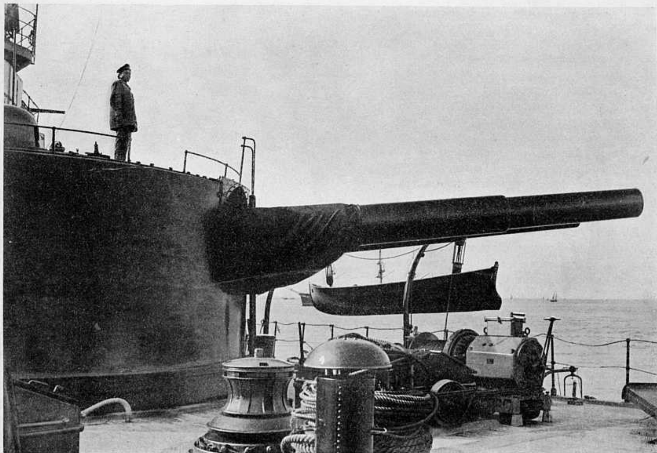
СОВРЕМЕННЫЙ БРОНЕНОСЕЦЪ (ТИПЪ «АЛЕКСАНДРА III»). БРОНЕВАЯ БАШНЯ СЪ ДВУМЯ ДВѢНАДЦАТИДУЙМОВЫМИ ОРУДИЯМИ. ДЛИНА ОРУДИЯ = 6,66 САЖ. = 12,2 МЕТР. ВѢСЪ ОРУДИЯ 59 ТОННЪ = 3,650 ПУД. ВѢСЪ СНАРЯДА НЕМНОГО БОЛѢЕ 20 ПУД. НАЧАЛЬНАЯ СКОРОСТЬ = 724 МЕТРА ВЪ СЕКУНДУ.
