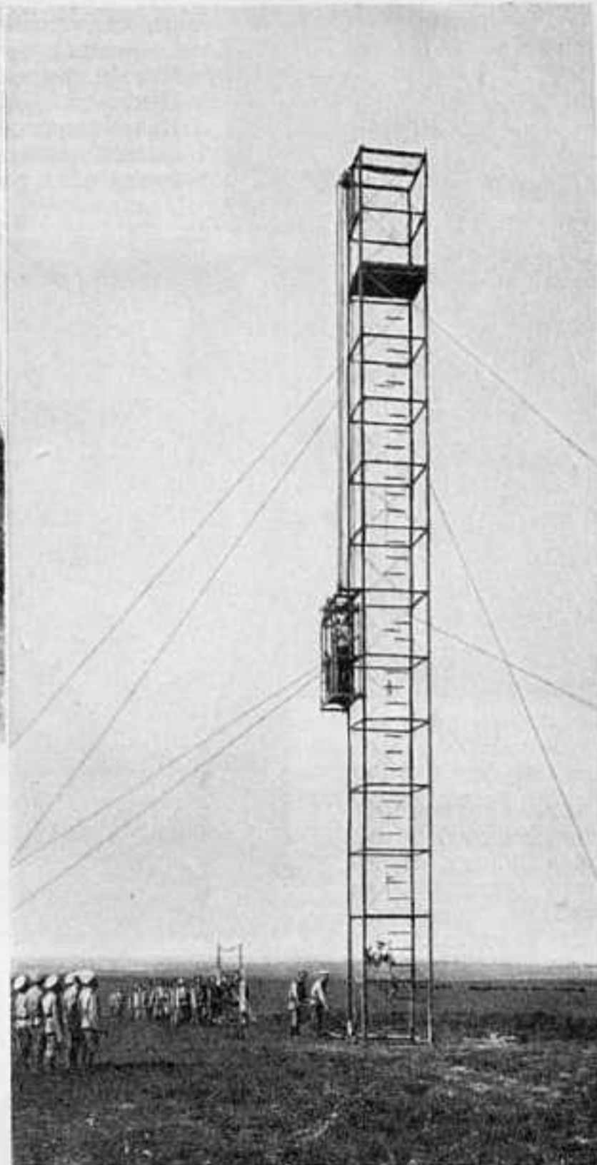
НАБЛЮДАТЕЛЬНАЯ ВЫШКА КАП. ДУБРОВСКАГО ВЪ УСТАНОВЛЕННОМЪ ВИДѢ. ИМѢЕТЪ 20 САЖ. ВЫСОТЫ. НАХОДИЛАСЬ НА ПОЗИЦИИ НА Р. ШАХЪ.
