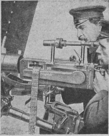
Новый тип германскаго пулемета.
