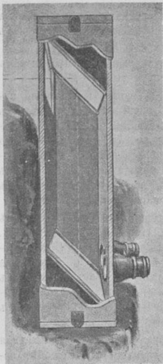
Перископъ въ разрѣзѣ.
