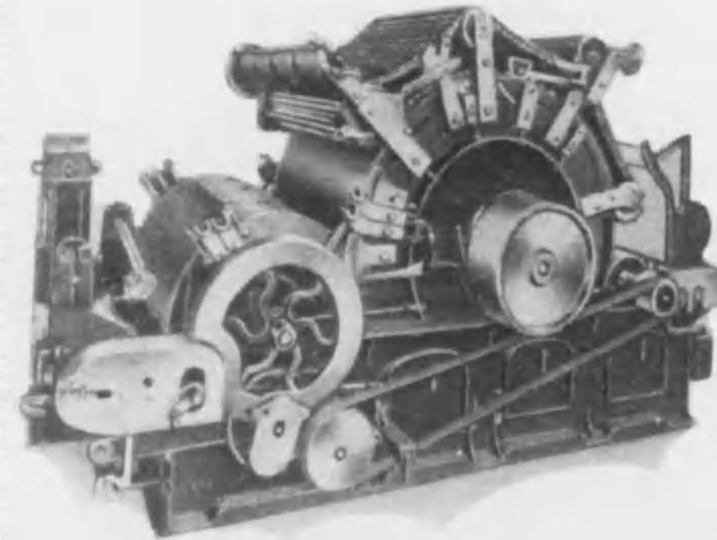
ブルツクスドキシ-會社 カーディング エンジン
