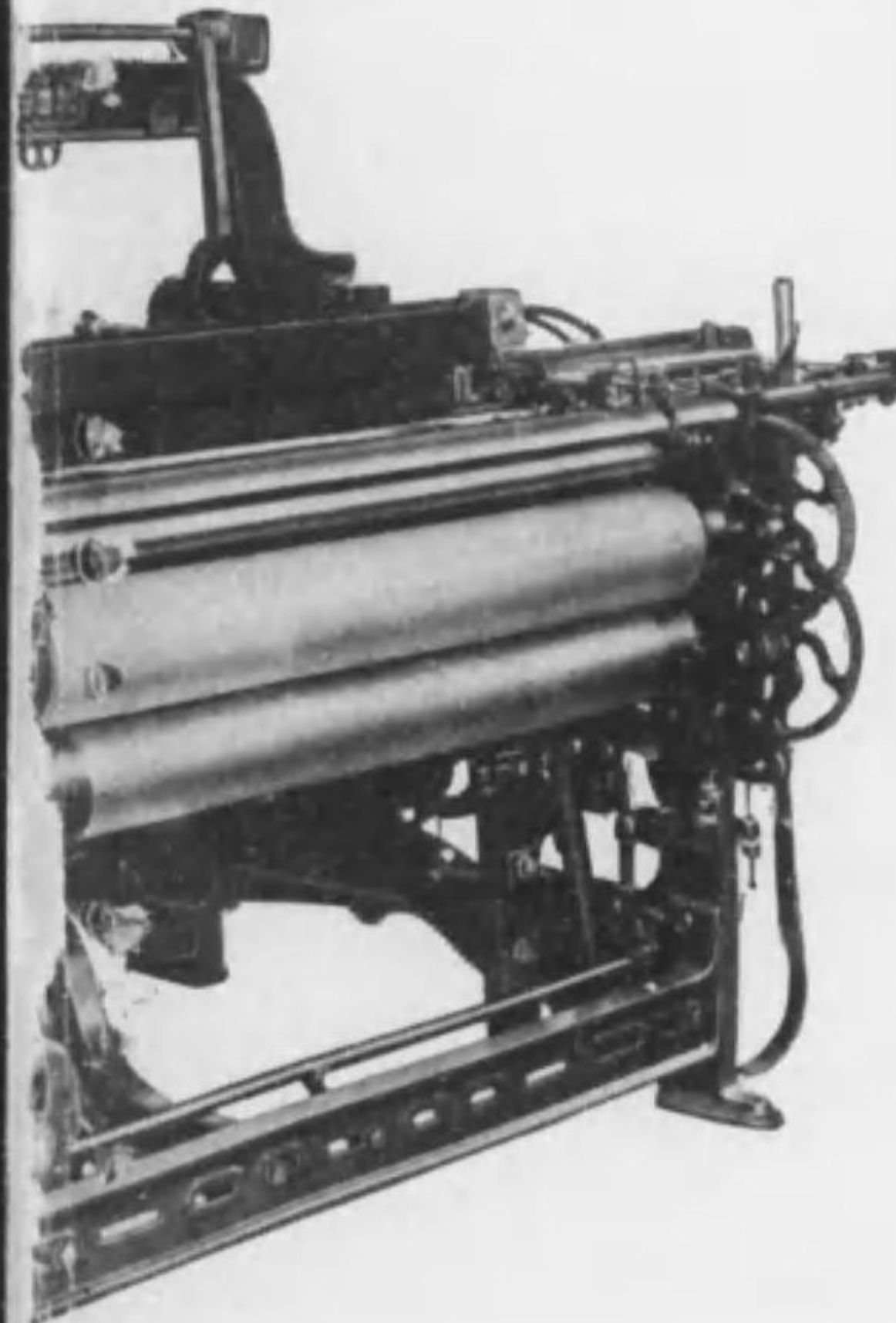
經糸切斷停止裝置
