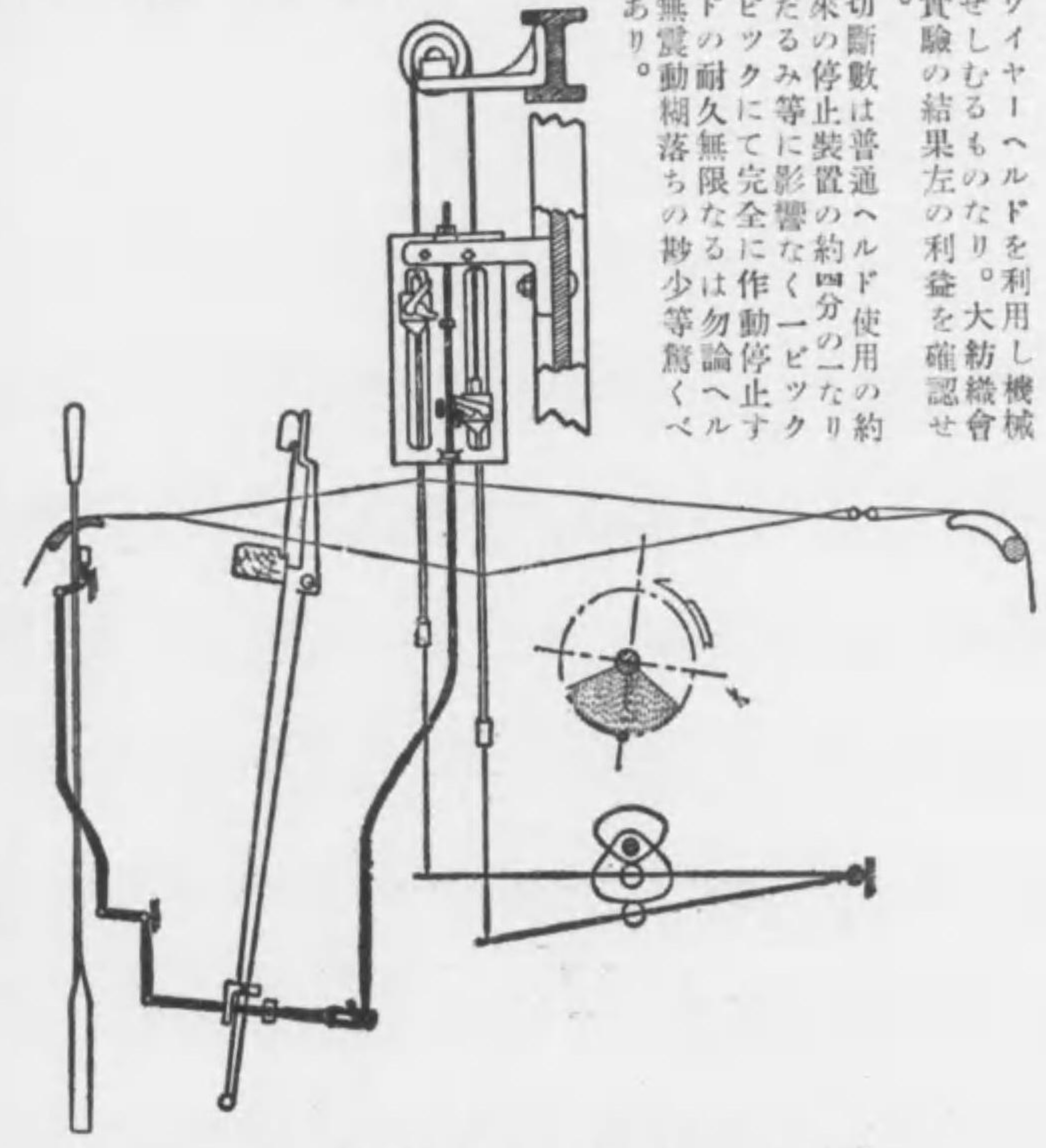
R.M.式經糸切斷停止裝置の聯動圖
