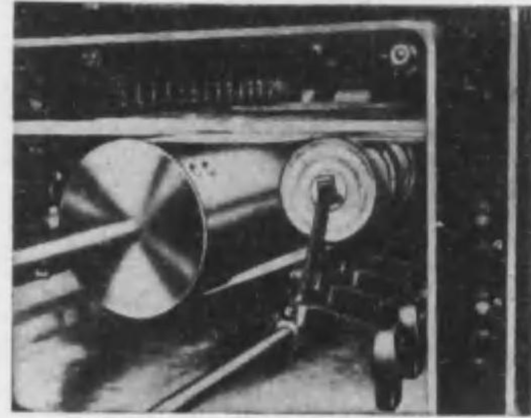
テープドライビング装置
