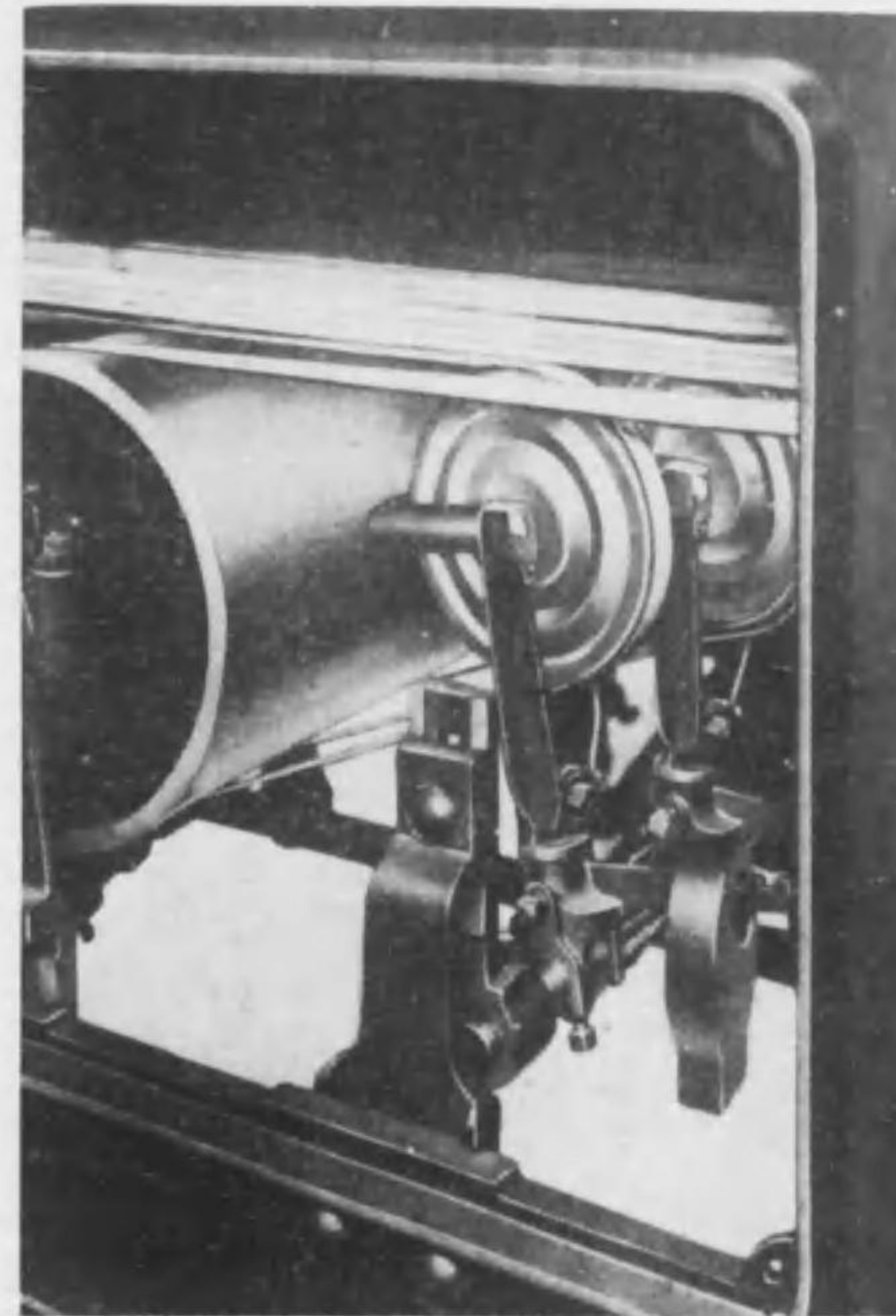
精紡機のチンローラー部
