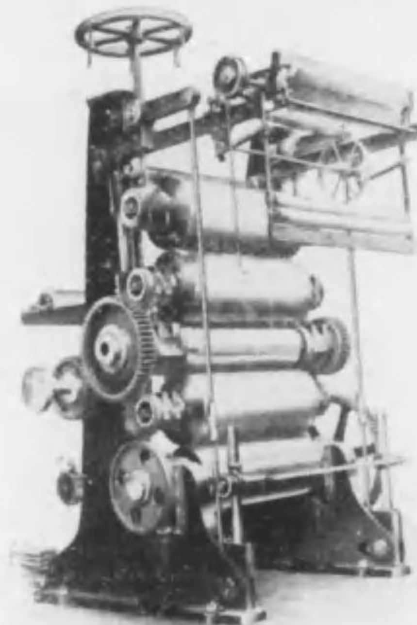
四本ロール製出カレンダー
