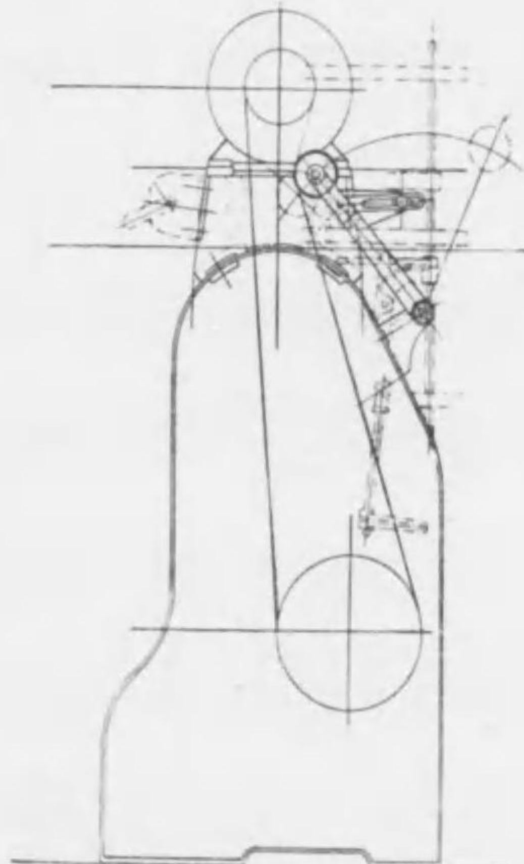
粗紡機用エリコンデバイス(特許出願中)
