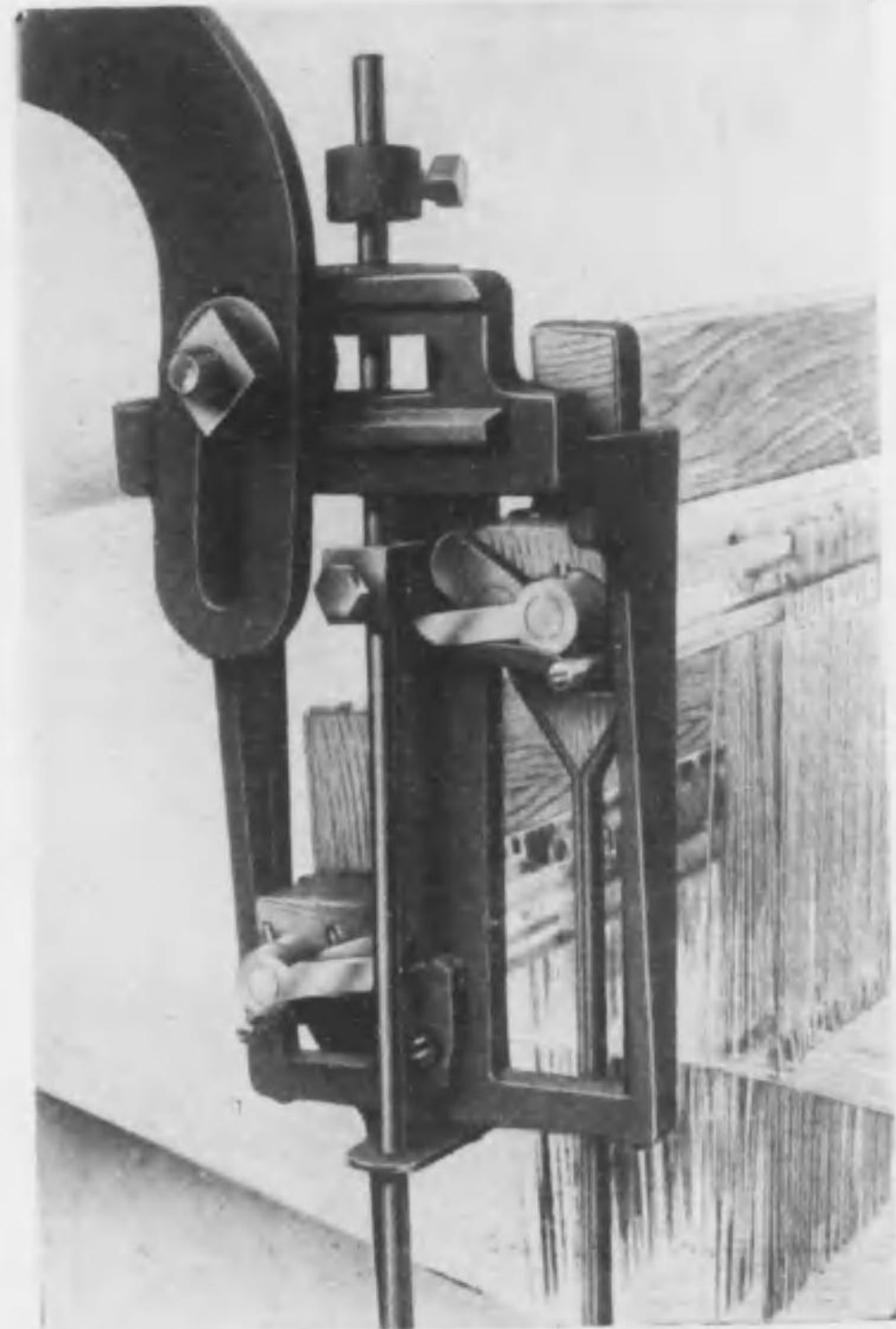
R.M.式經糸切斷停止裝置側面(停止運動を起したる場合)
