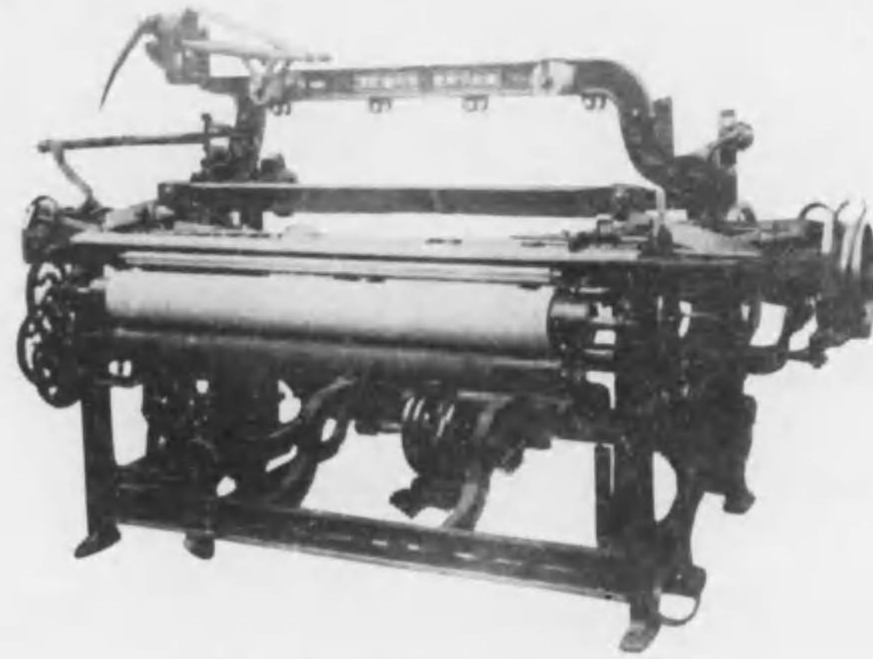
豊田式“N”式上打織機
