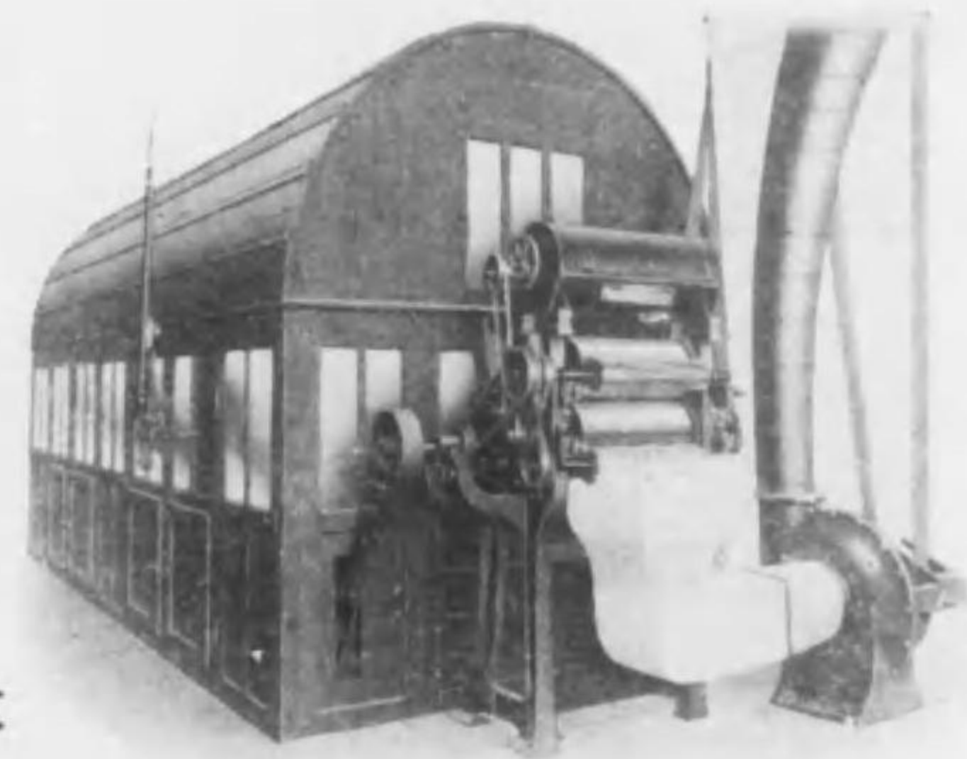
機毛乾式風熱
