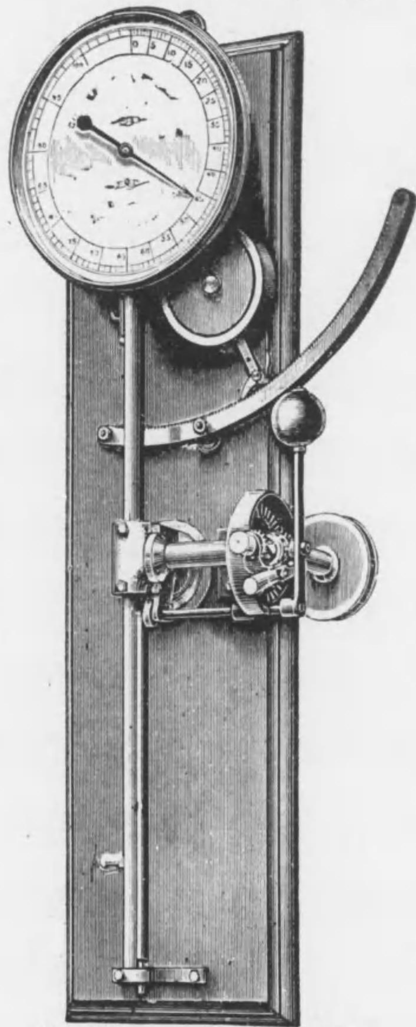
Fig. E122 AUTOMATIC YARN TESTER
