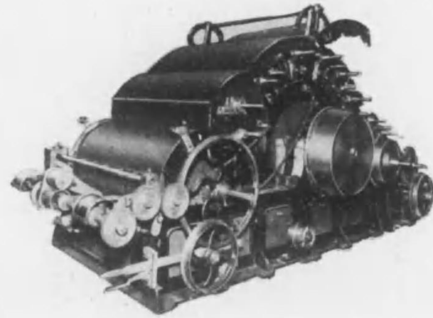
梳毛機
