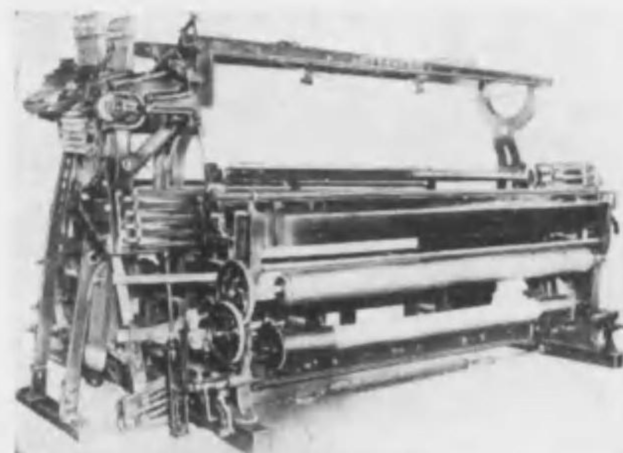
S型四幅毛織機
