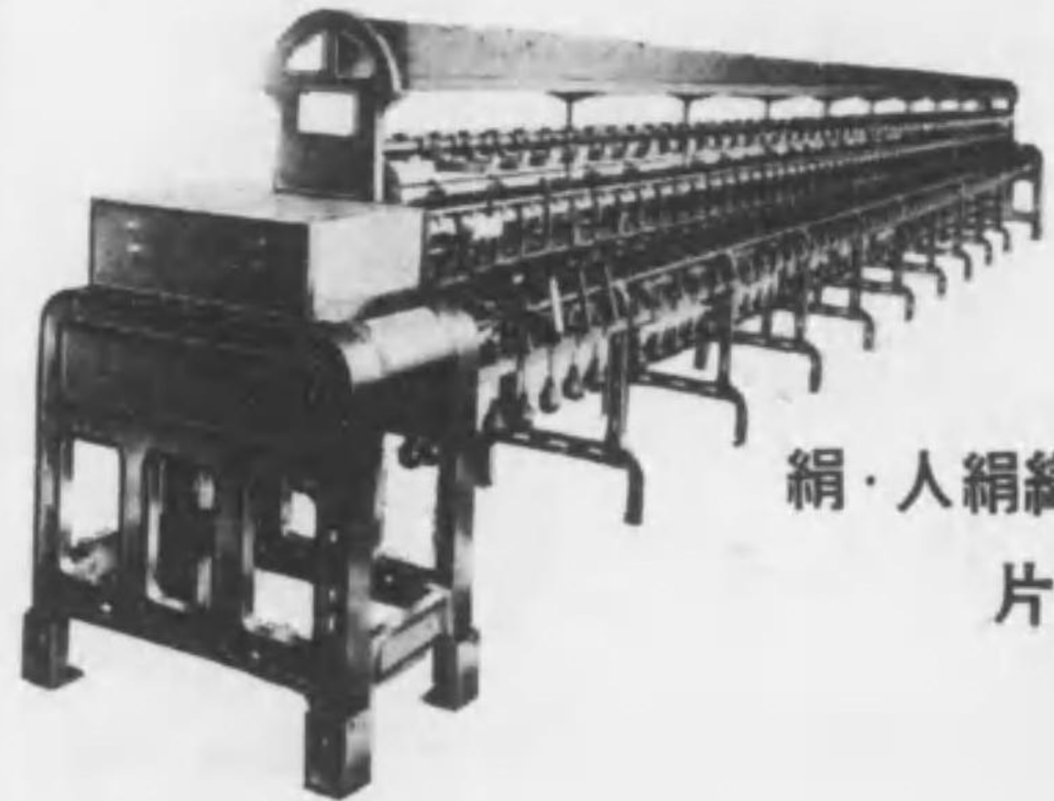
クイツク トラバース ワインダー
