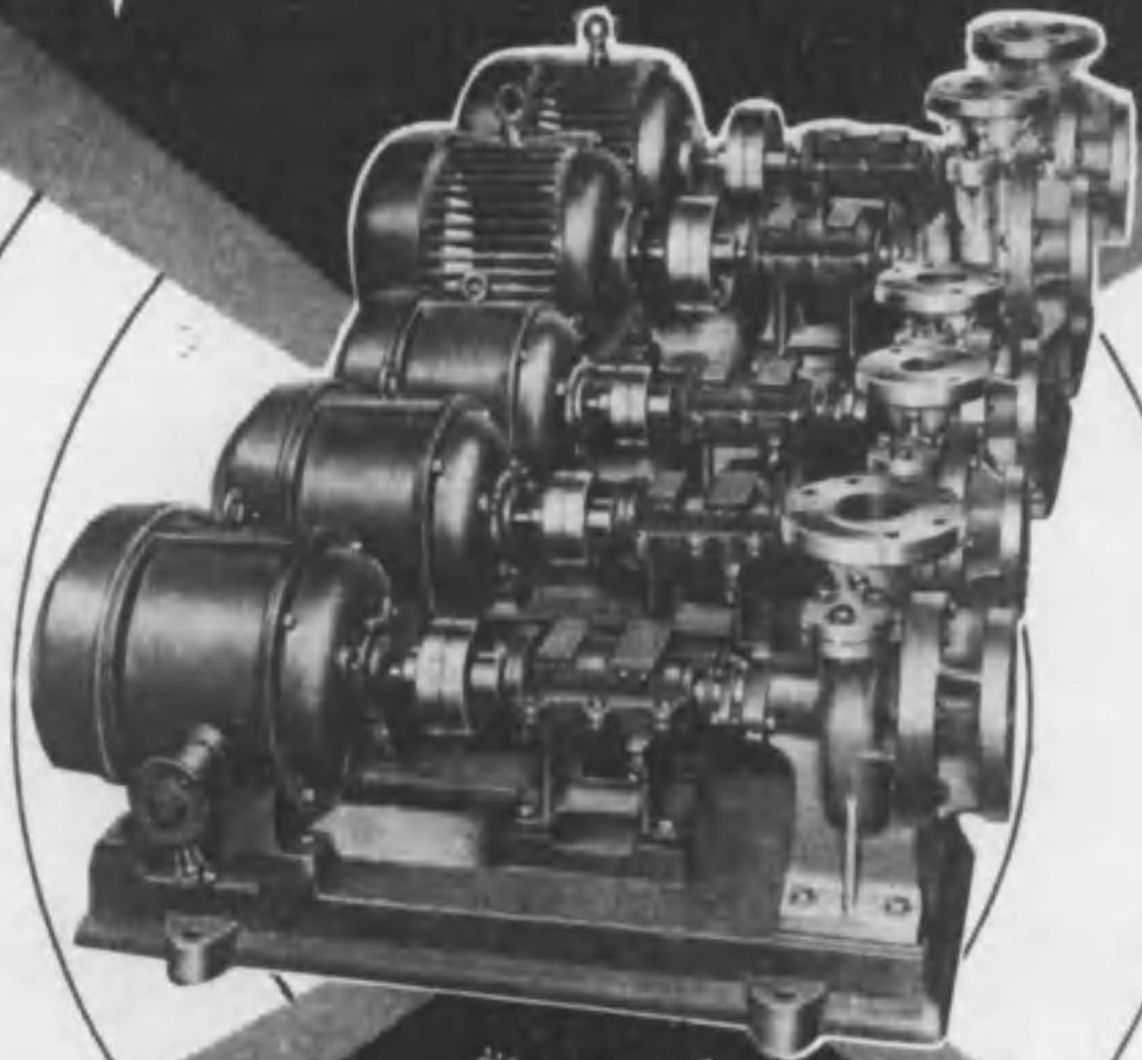
硬鉛製耐酸ポンプ
