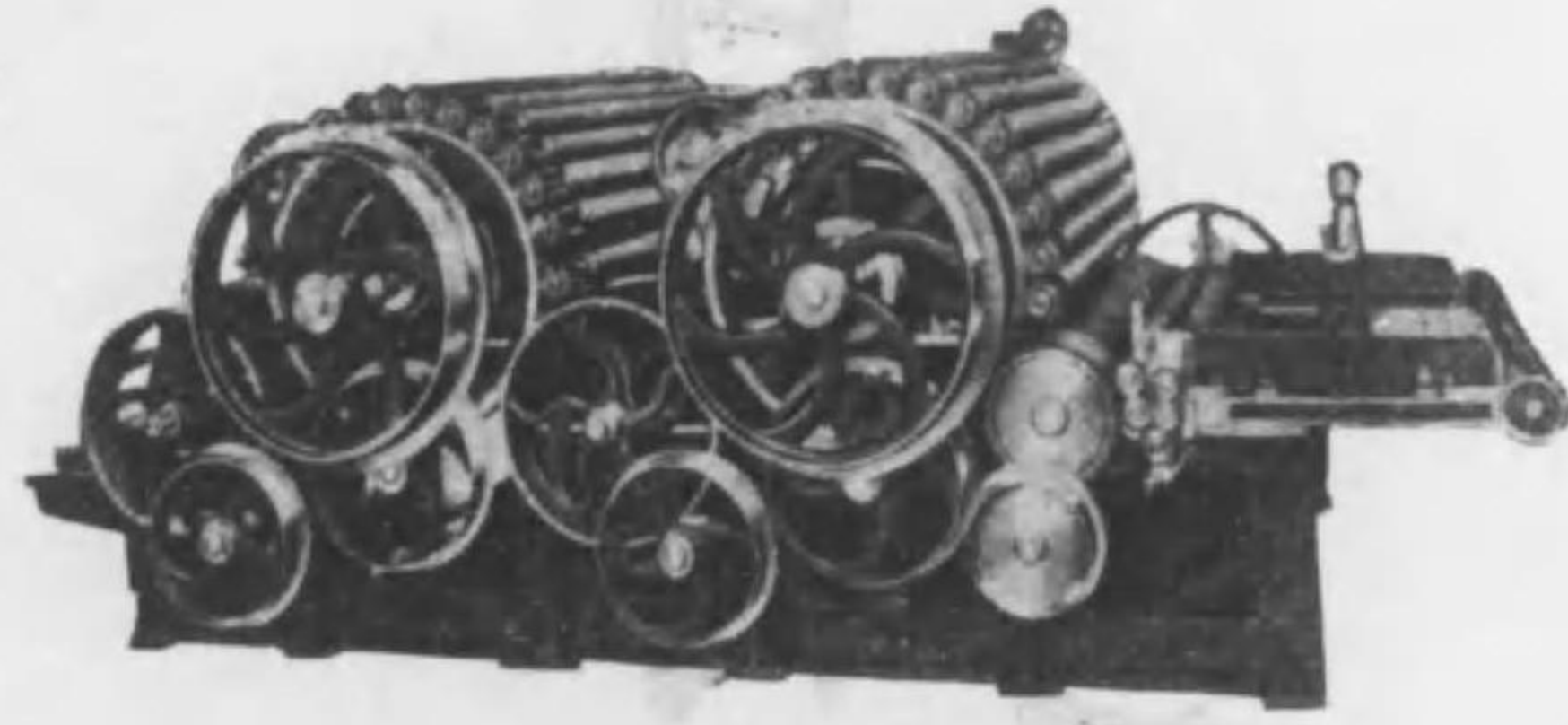
シユワルベ型 紡毛カード
