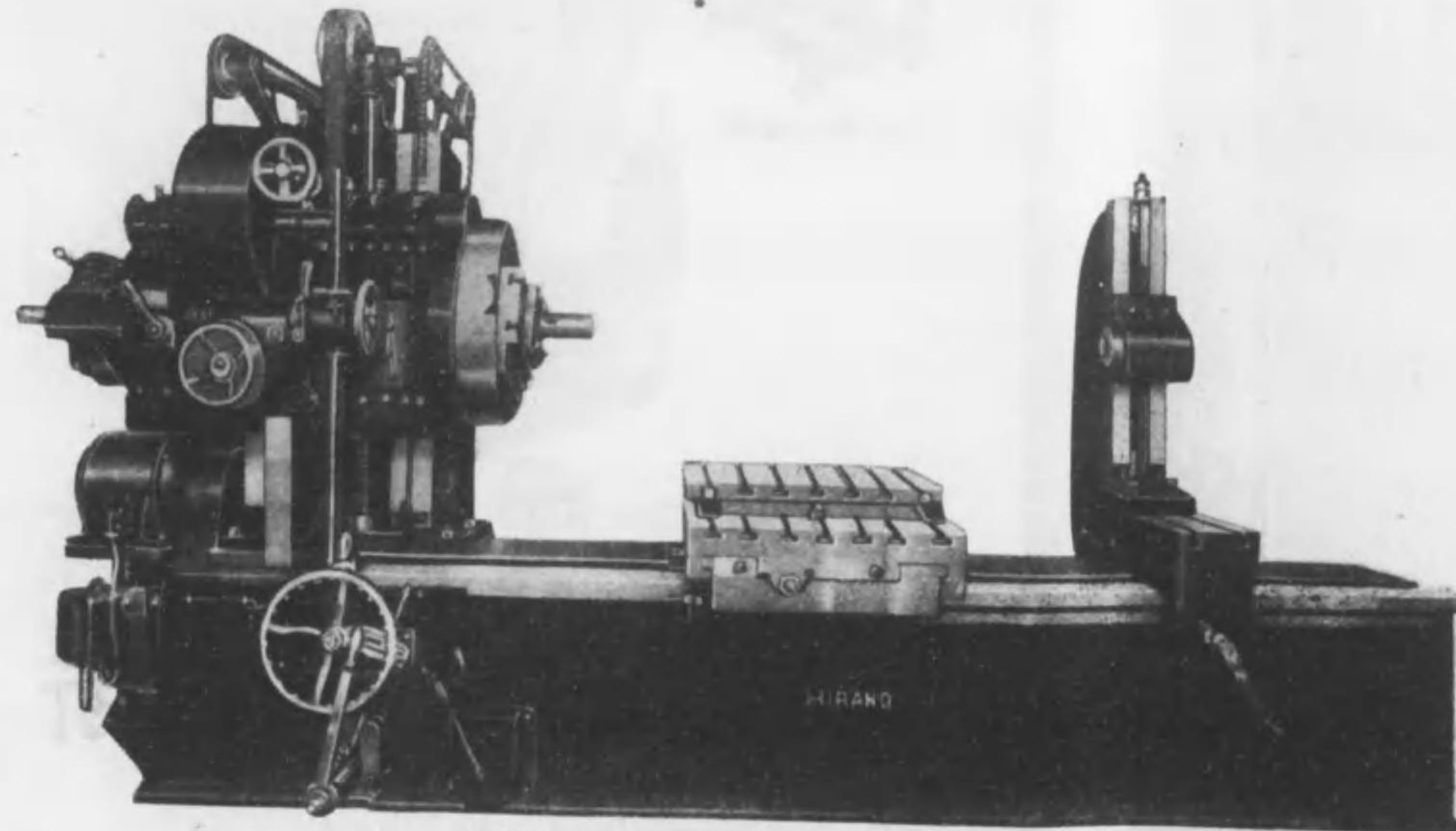
HSB型四番中グリ盤
