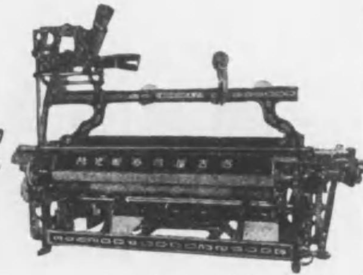
四丁Dビーム付織機
