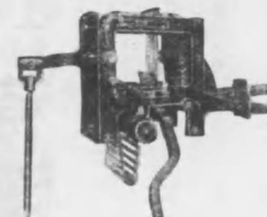
普通ドビー装置
