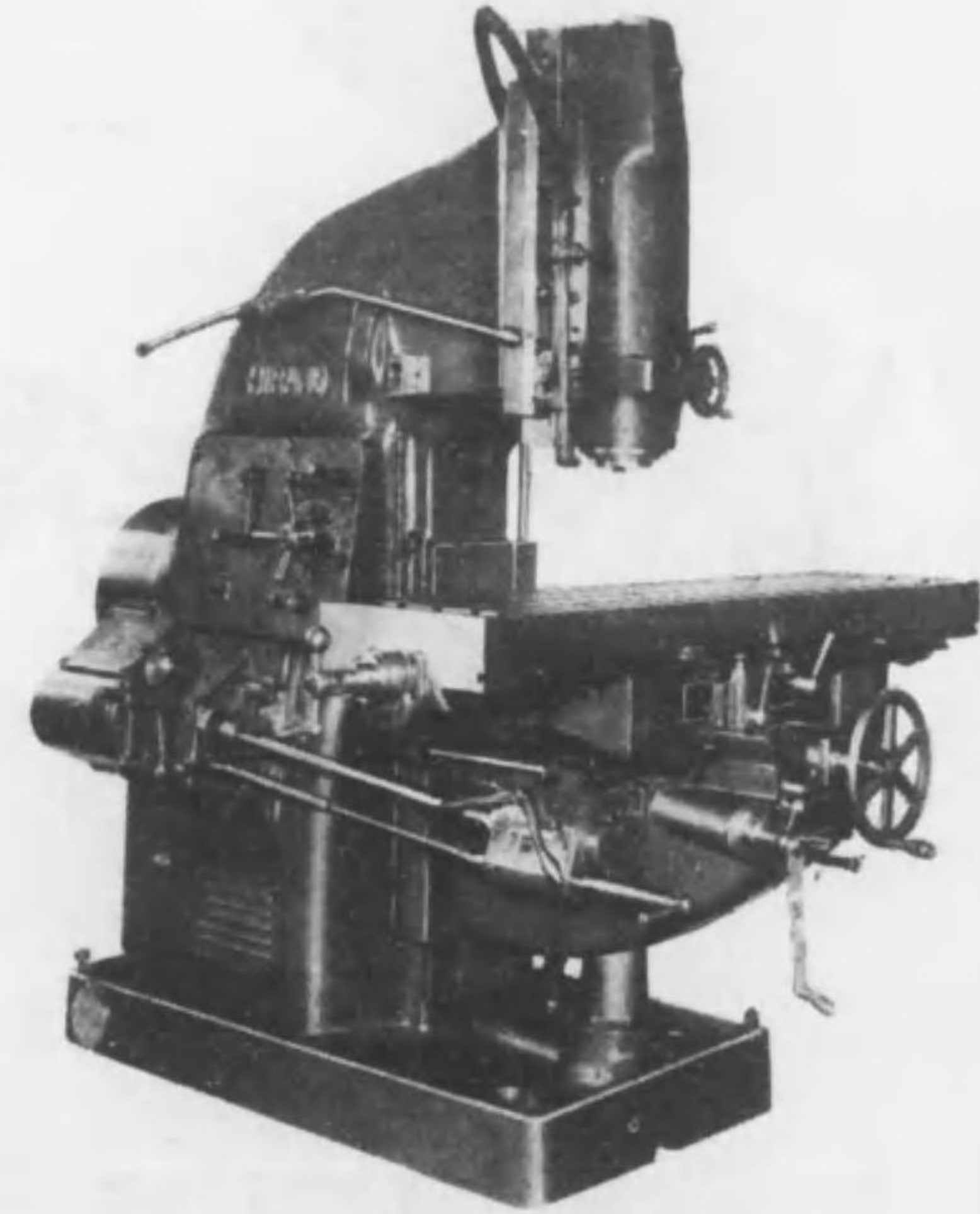
VCM型四番竖フライス盤
