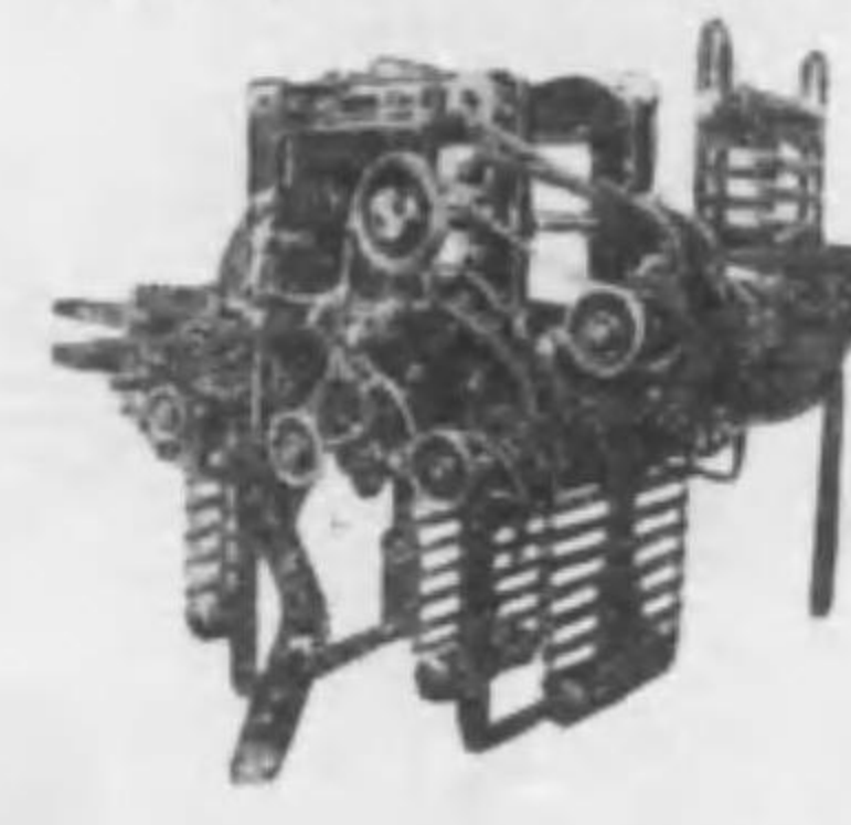
普通ドビー装置
