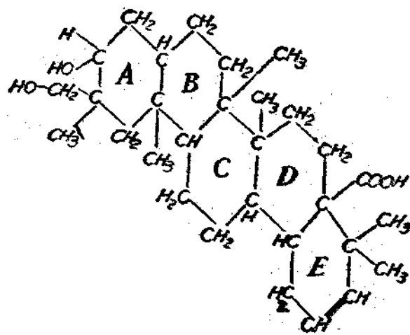
(IX) Hederagenin
