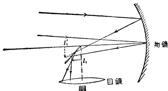
圖 8 . 反射望遠鏡
