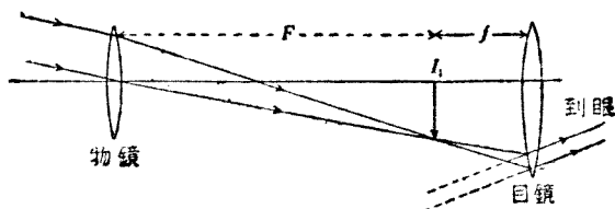
圖 78. 正常調準的天文望遠鏡
