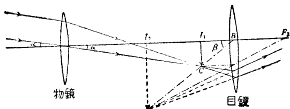
圖 77. 天文望遠鏡
