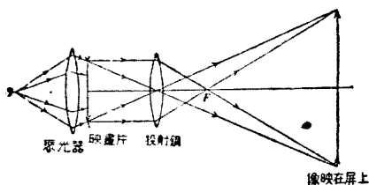
圖 30. 幻燈
