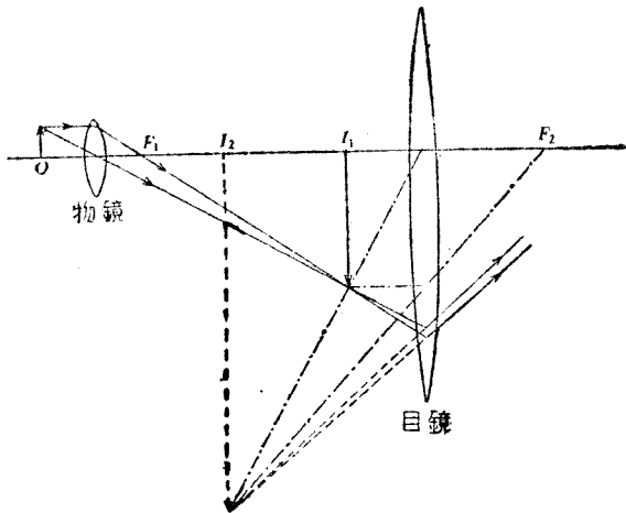
圖 75. 複式顯微鏡
