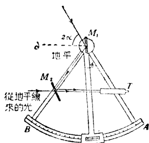
圖 9. 六分儀
