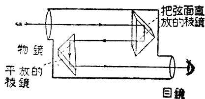
圖 80. 稜鏡雙眼望遠鏡
