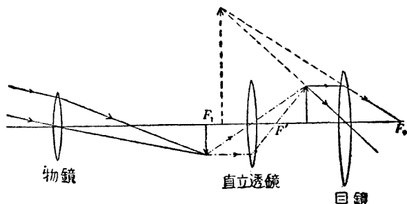
圖 79. 地上望遠鏡
