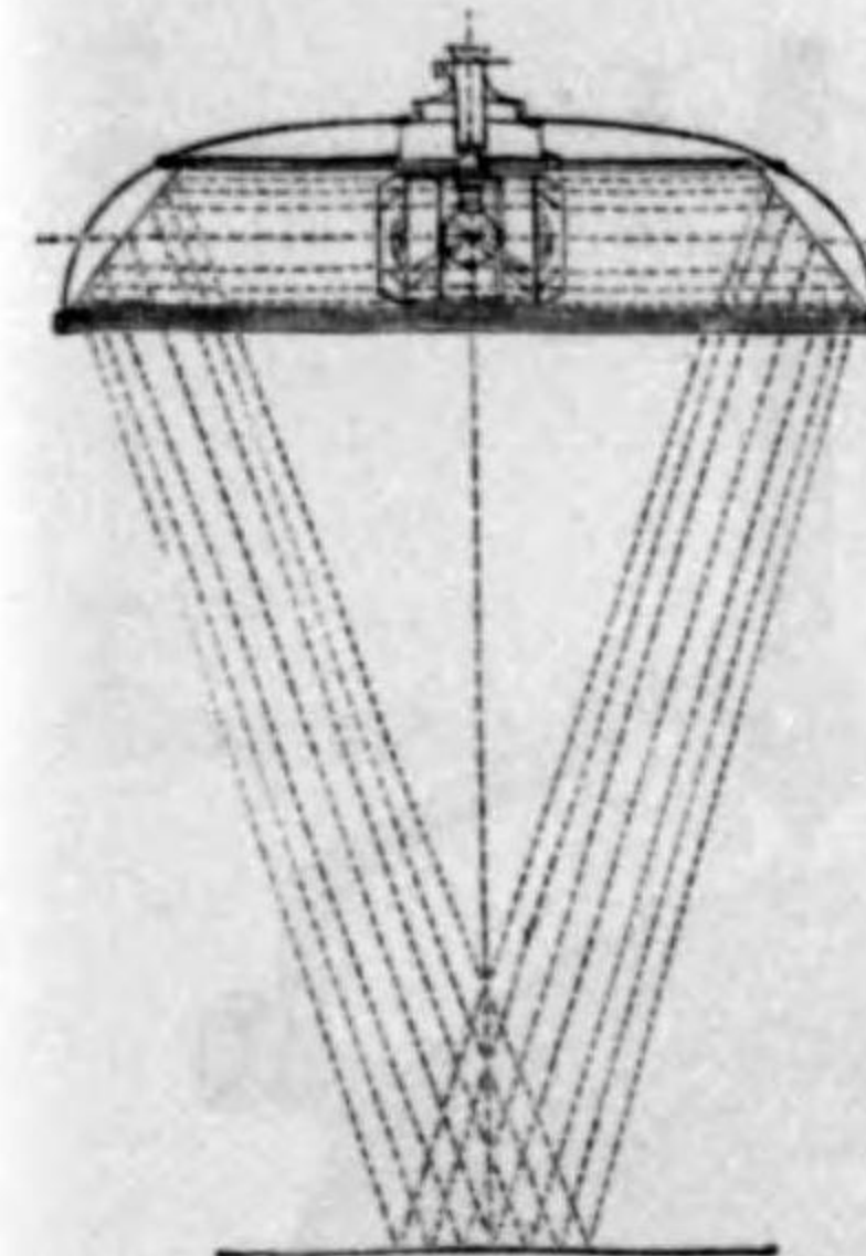
(シアリテーク無影照明燈ノ原理ヲ示ス)
