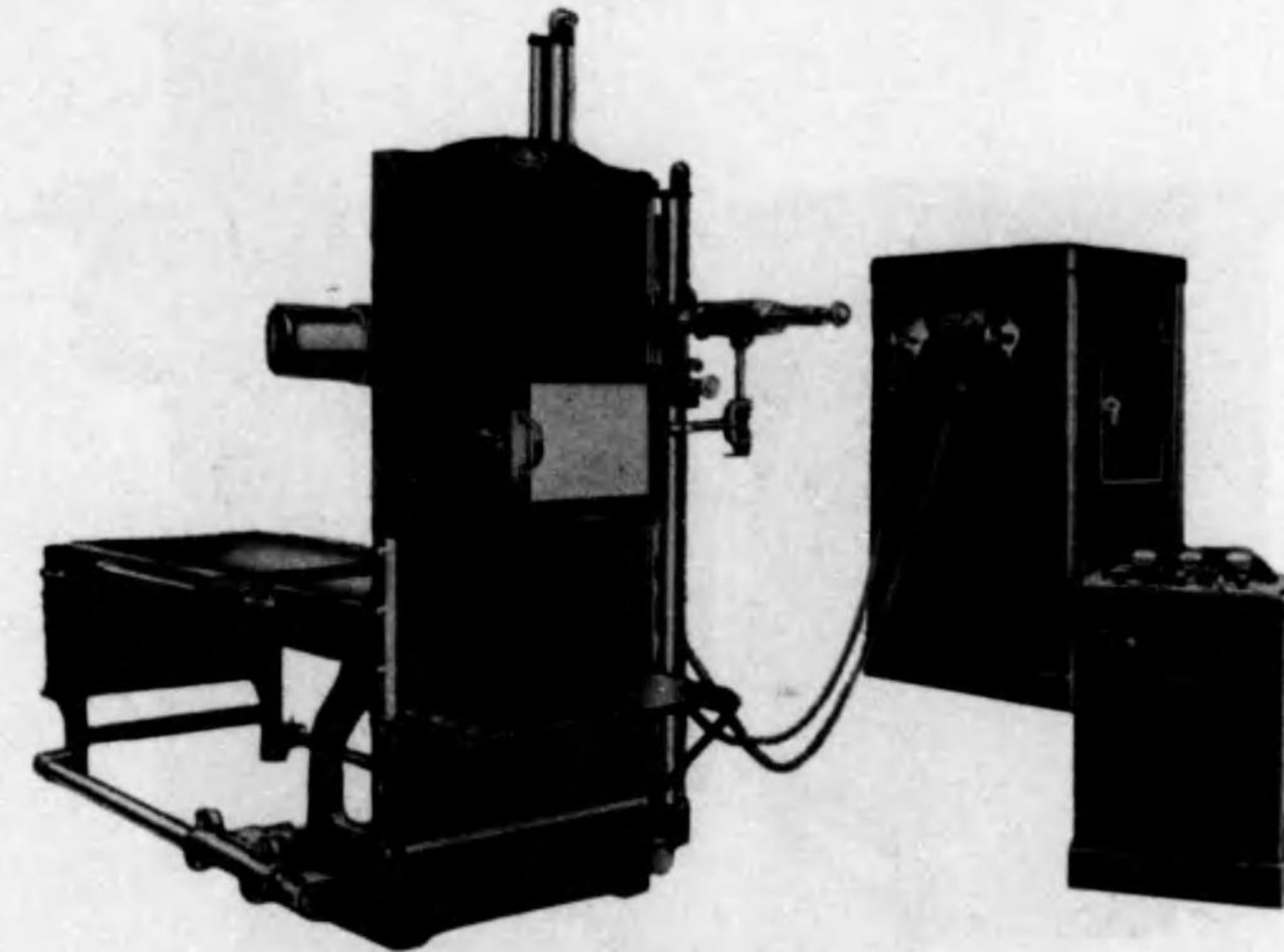
No. O 40 Yen 4,000.00 レントゲン装置 八雲號
