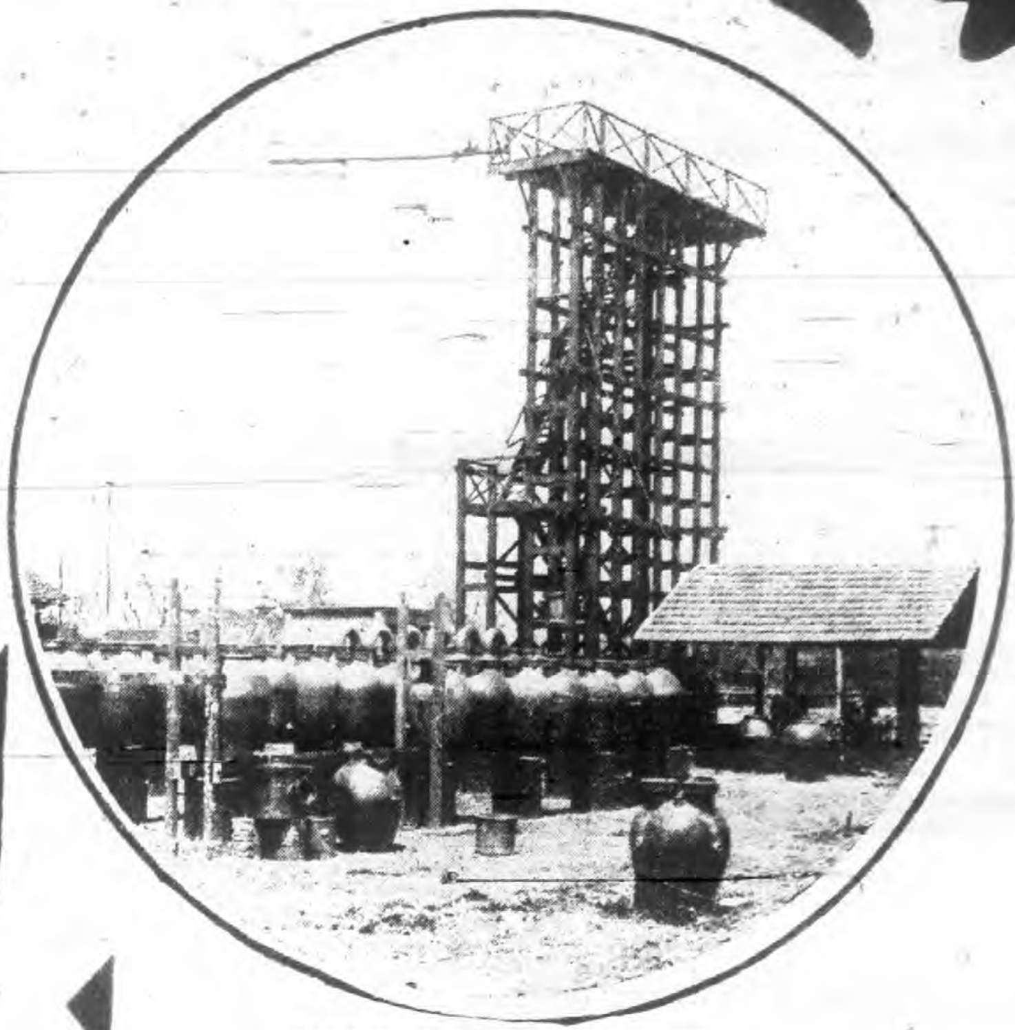
影攝塔酸鹽之廠化電原天
