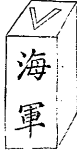
三角點標石(甲)
