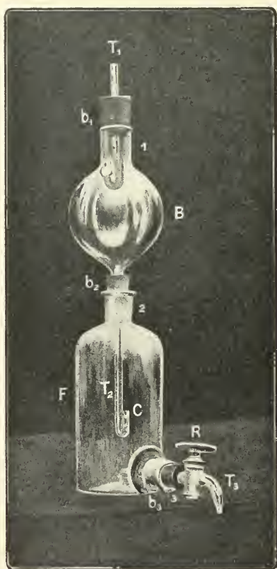
FIG. 236.—Radiogene. (Siemens.)
