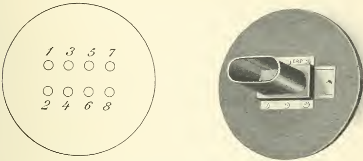
FIG. 56.—Walter's radiometer. (Siemens.)
