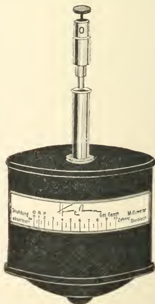
FIG. 55.—Bauer qualimeter. (Favre.)
