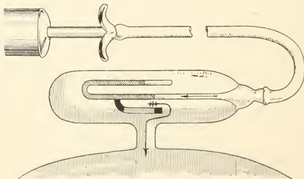
FIG. 41.—Bauer air-valve. (Favre.)
