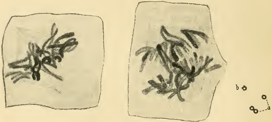
Fig. 1. 16 gesplattene Chromosomen. Metaphase. Fig. 2. Anaphase. In jedem Tochterkern 16 einfache Chromosomen. Fig. 3. Chromosomenquerschnitte. a in der Metaphase, b in der Anaphase.
