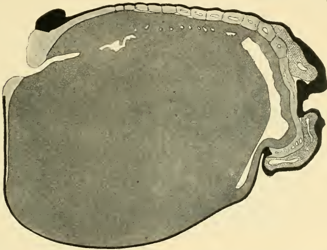
Fig. 9a. Kombinierte Zeichnung zweier paramedianen Schnitte des Eies \times 30 ( \frac{1}{2} ). Schwarz Hautektoderm, doppelt schraffiert Gehirnanlage, dunkelgrau Entoderm, hellgrau Mesoderm.
