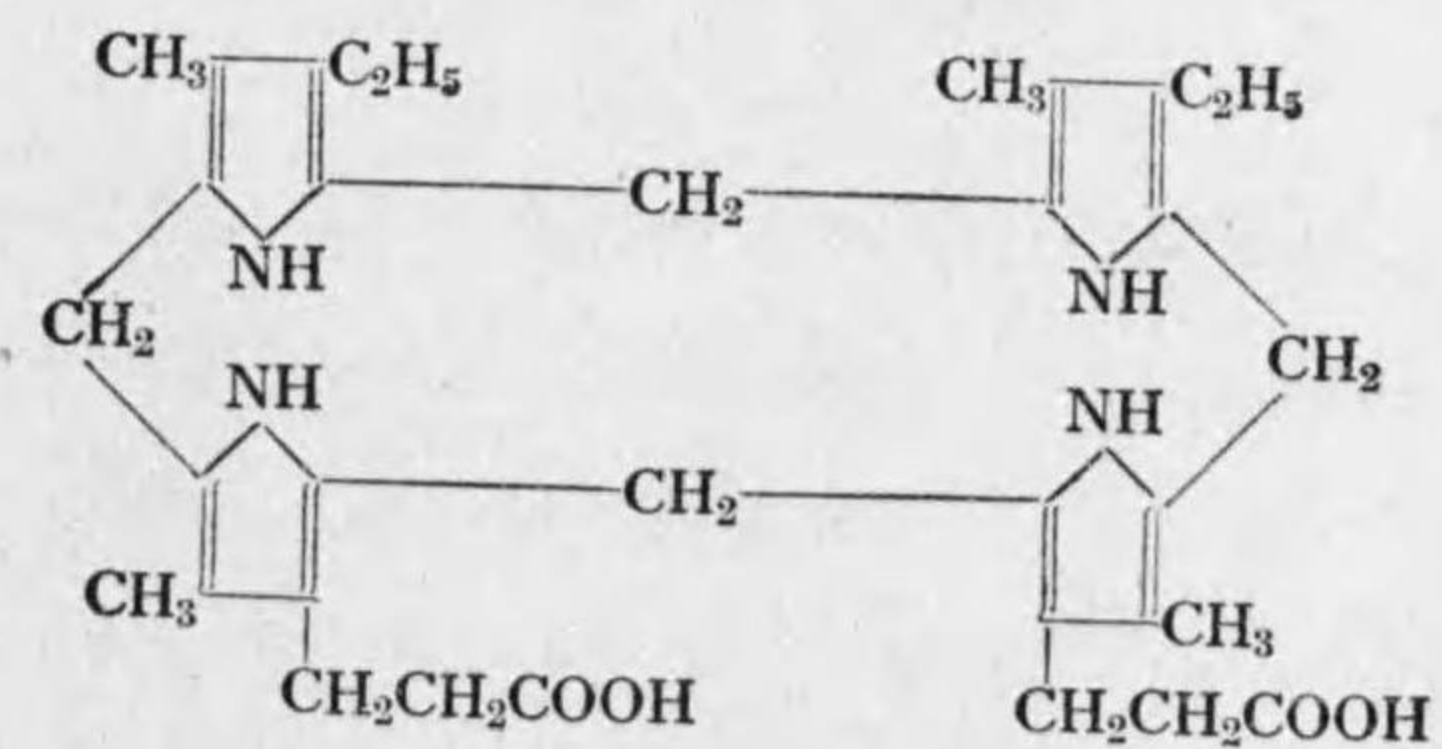
Mesoporphyrinogen C 34 H 44 N 4 O 4
