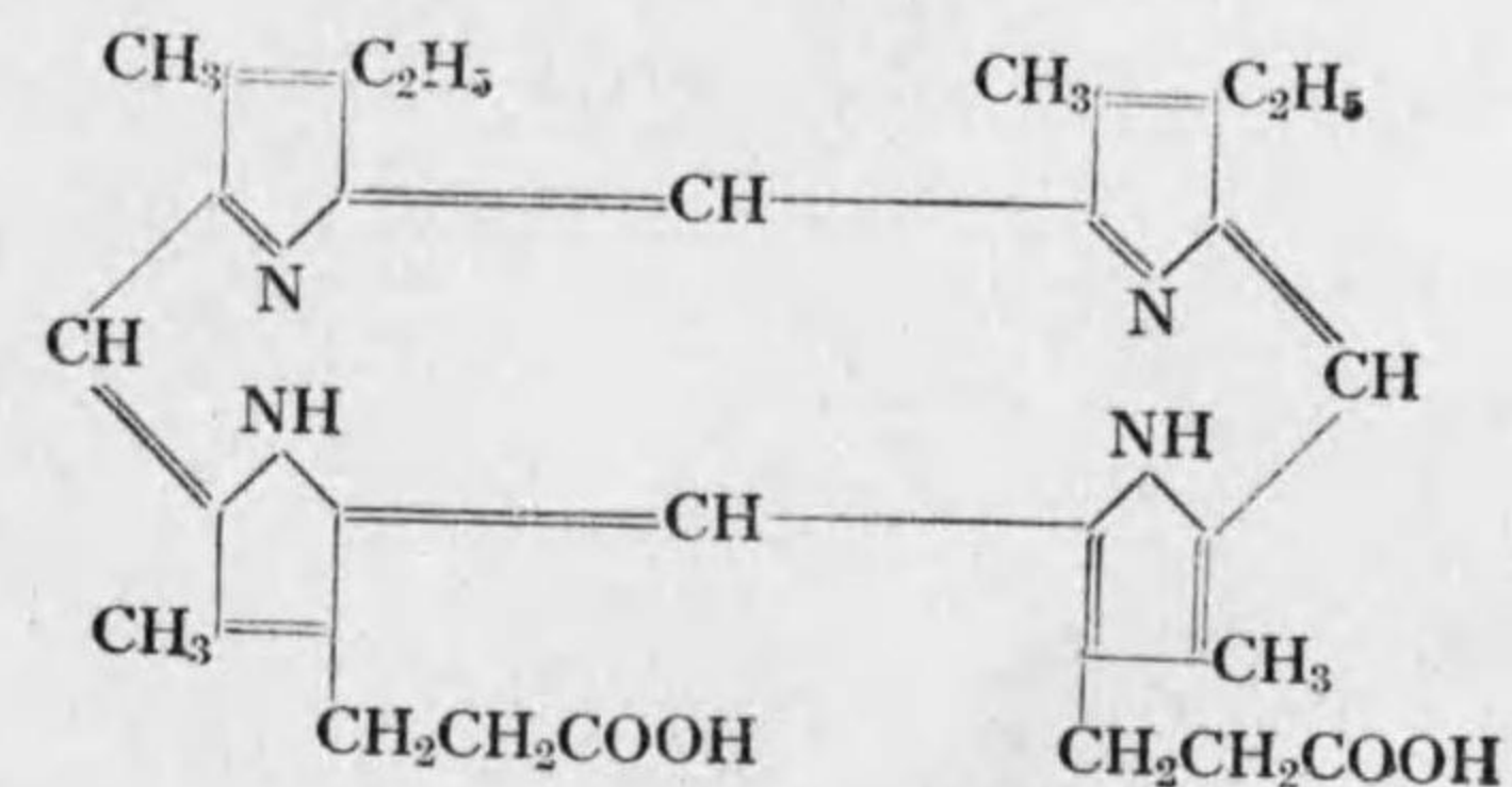
Mesoporphyrin C 34 H 38 N 4 O 4
