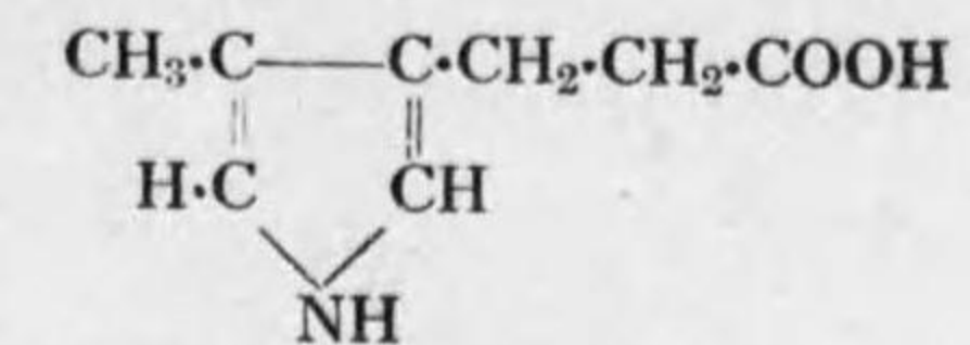
8. Opsopyrrol-炭素酸
