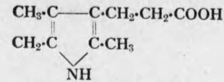
7. Phyllopyrrol-炭素酸
