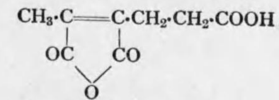
Hematin-酸-失水物
