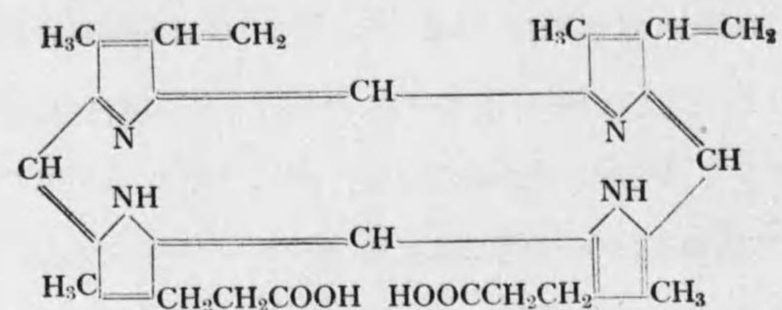
Protoporphyrin C 34 H 34 N 4 O 4
