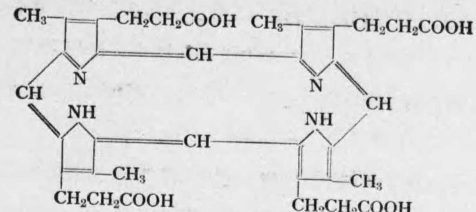
Koproporphyrin
