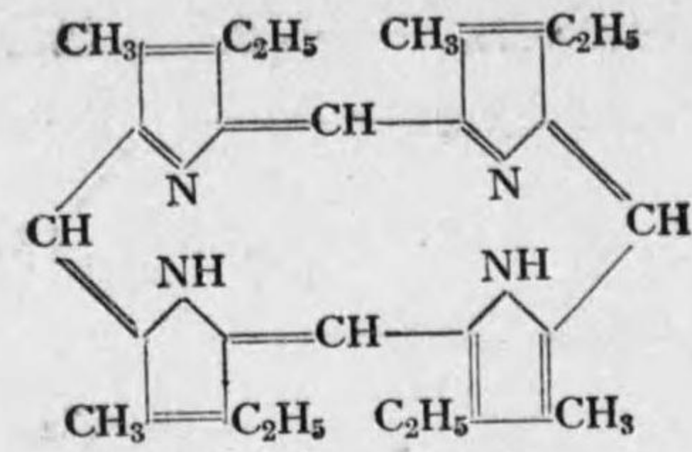
Aetioporphyrin C 32 H 38 N 4
