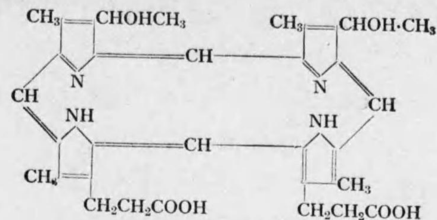
Hematoporphyrin C 34 H 38 N 4 O 6
