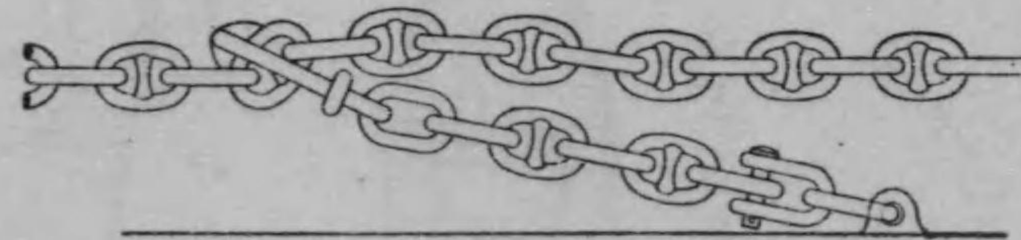
チェインスリッパ ストッパー
