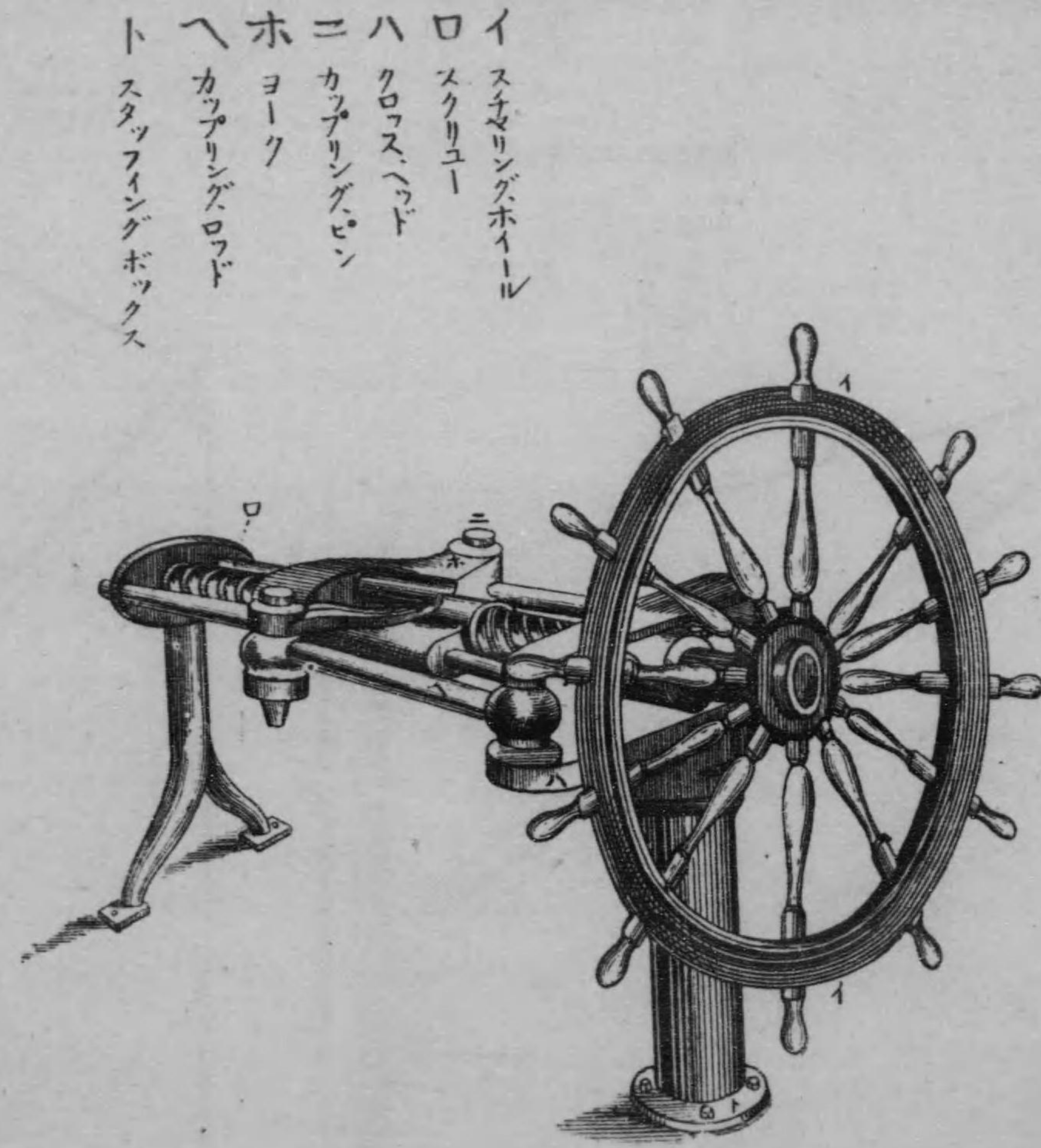
第三十九圖 手用操舵機及レリービングブテークル
