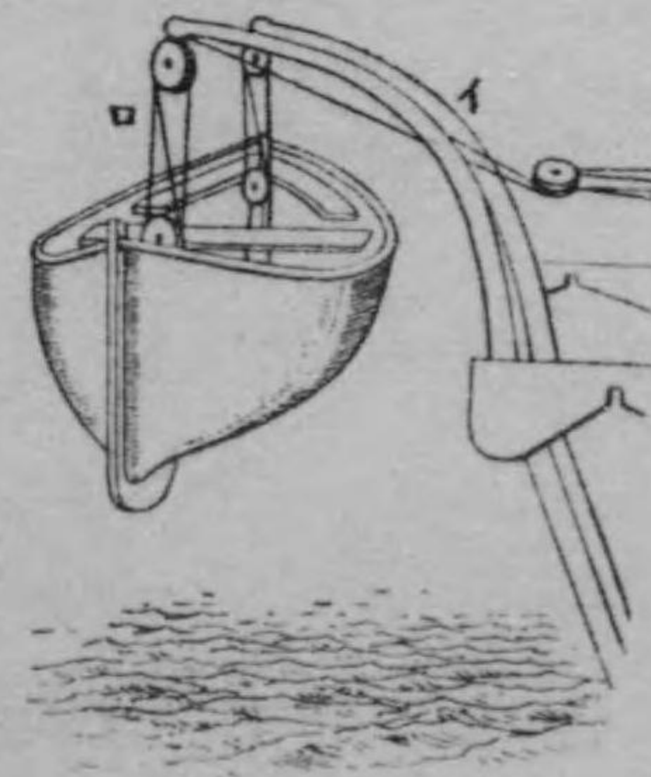
イ ホートゲベツト ロ ホートテークル
