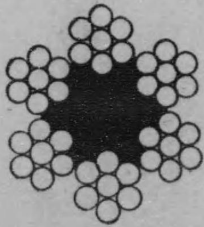
インフレキシブルスチールワイヤロープ
