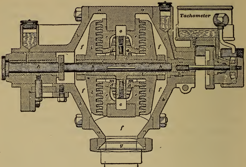
FIG. 43.—DOW TURBINE.
