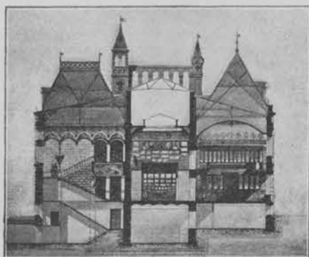
Домъ Петра Ивановича Щукина на Прѣснѣ, въ Москвѣ, Проектир. и постр. архит. А. Э. Эриксонъ. (Фасадъ, разрѣзъ и планы).
