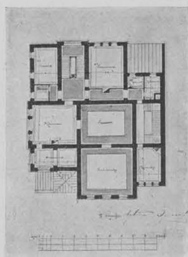
Домъ Петра Ивановича Щукина на Прѣснѣ, въ Москвѣ, Проектир. и постр. архит. А. Э. Эриксонъ. (Фасадъ, разрѣзъ и планы).
