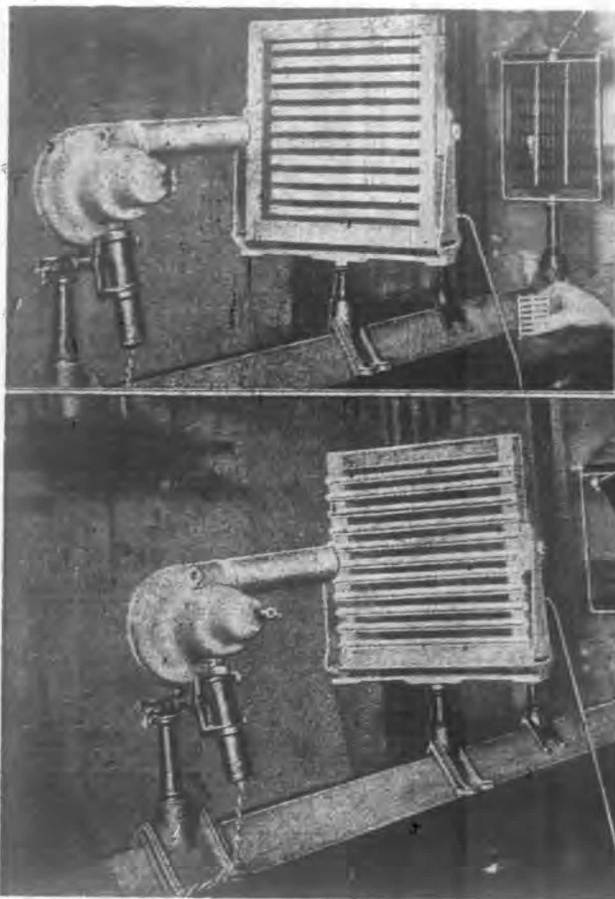
(上)表示圓棍之後風葉離靜止之態 (左上) 表示扁木柵後風葉不為動
