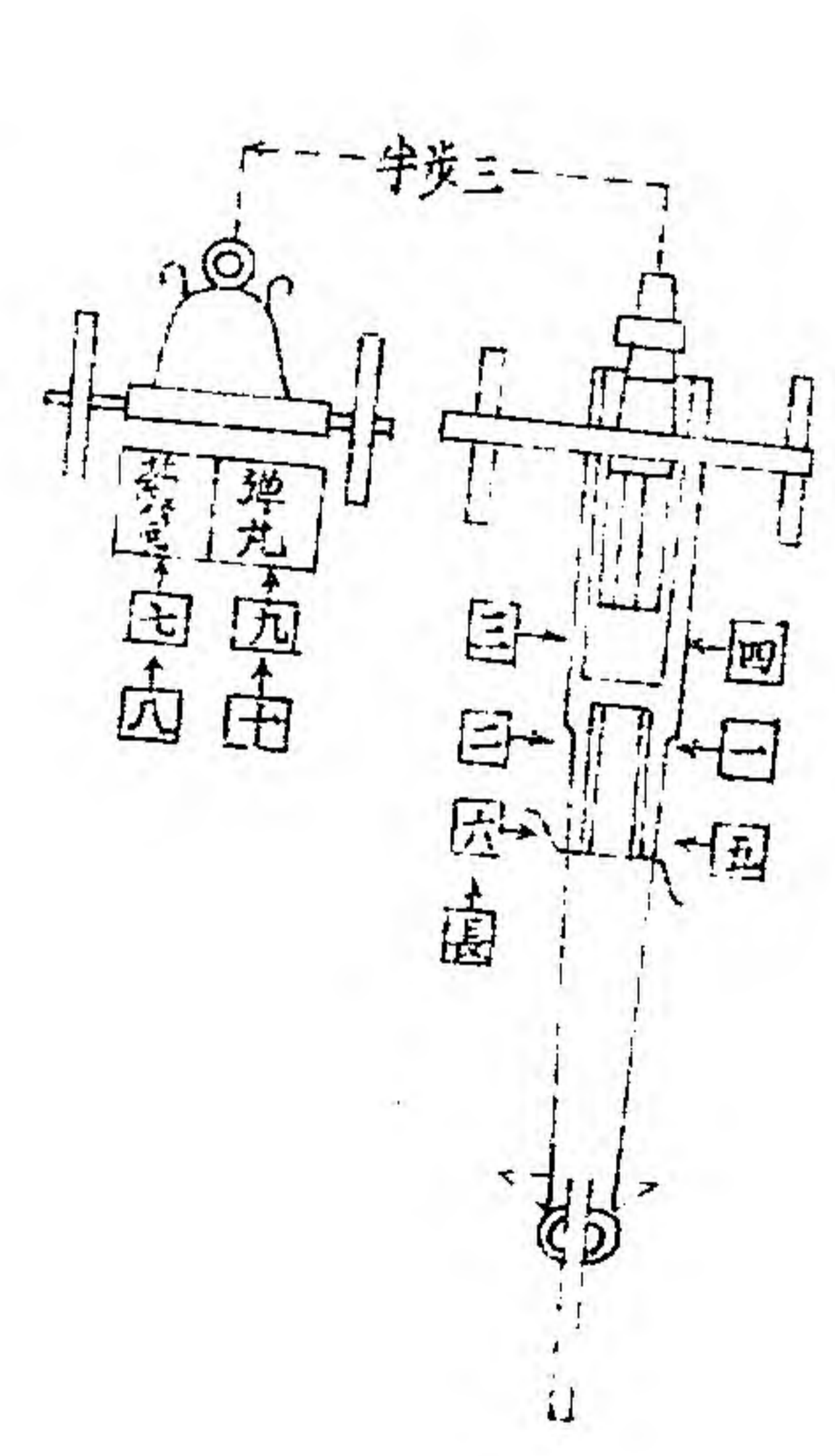
11 四年式十五榴(放列)
