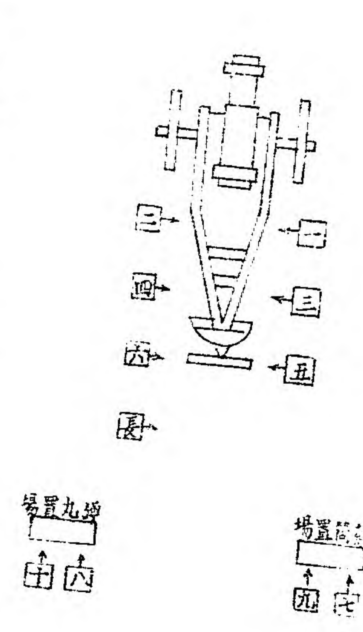
13 三八式十加(放列)
