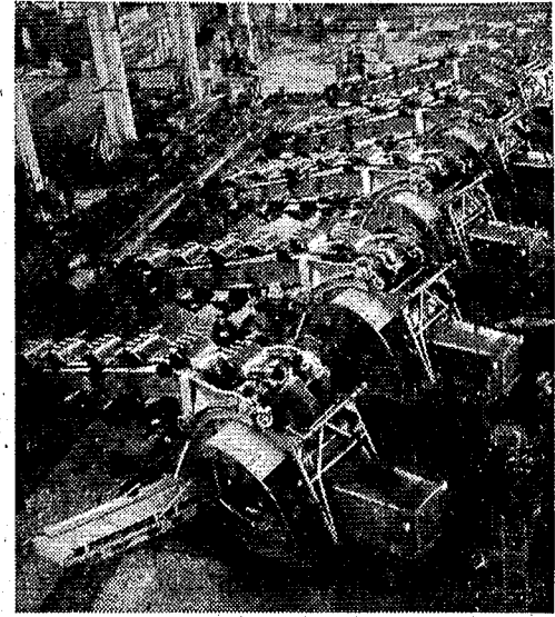
上海水工机械厂今年成批投入生产的新产品——大型挖沟机。它挖沟的宽度，最宽可达三米二，底部深一米一，最深最深达三米三。
