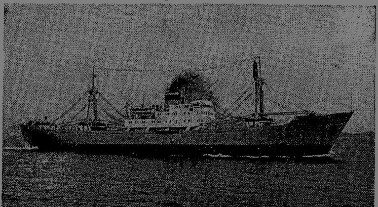
大連造船廠建造的名為「首領」的新型 遠洋貨輪，是我國自行設計和建造的，遠洋載重 量為六千噸，排水量為八千九百噸，續航力為七 千五百海里。(劉增輝攝 新華社稿)
