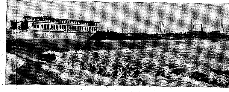
我国又一座规模巨大的电力抽水站——建在长江与京杭大运河交汇处附近的江都水利枢纽工程第二抽水站,于一九六四年八月下旬建成,并已试运转。这座水利枢纽工程的设计、施工、设备制造和安装等工作,都是依靠我国自己的技术力量进行的。这是江都水利枢纽工程第二抽水站外景。
