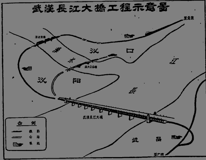
↑ 武漢長江大橋全部工程示意圖。
