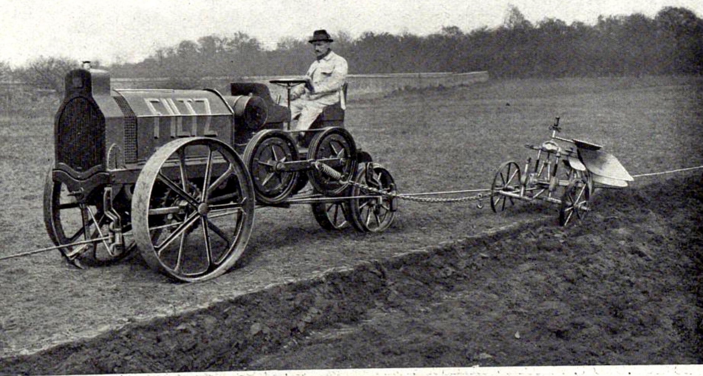
LE TRACTEUR-TOUEUR FILTZ GRIVOLAS EN TRAVAIL A SAINT-GERMAIN, SE HALANT SUR SON CABLE, ET TIRANT UNE CHARRUE BRABANT DOUBLE.
