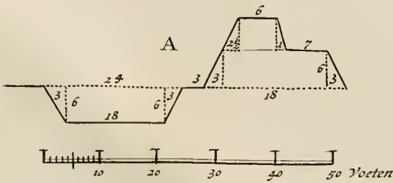
A F B E E L D I N G V A N D E L E G E R A . Profiel van de Engelsche Schans . C . Profiel van de Vriesche Schans . B . Profiel van de Hollandfche Schans . D . Redout .
