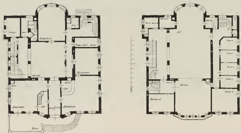
ARCHITEKTEN SCHILLING & GRAEBNER-DRESDEN Ratskeller in Schwarzenberg, Erzgeb.: Gesamtansicht und Grundrisse
