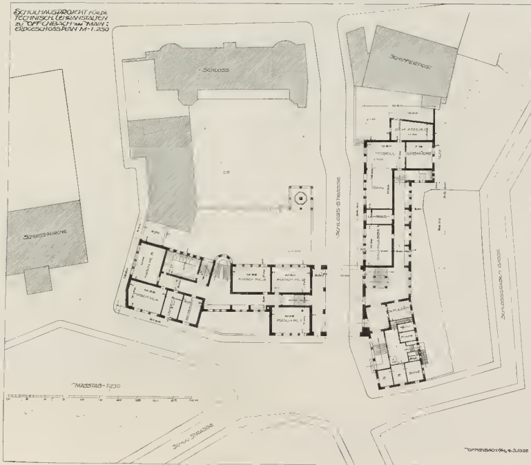
HUGO EBERHARDT-OFFENBACH a. M. Schulhausprojekt für die technischen Lehranstalten in Offenbach a. M.
