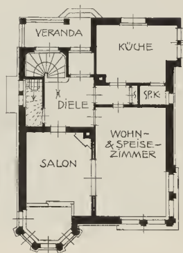
Grundrisse der Häuser Wolf in Heidelberg, Lutz in Saarburg, des Doppelwohnhauses und des Hauses Loewenich in Heidelberg
