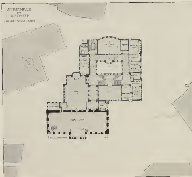
ARCHITEKT FRITZ SCHUMACHER-DRESDEN Stadthaus für Bremen (Engerer Wettbewerb), Grundrisse des Erdgeschosses und Hauptgeschoss
