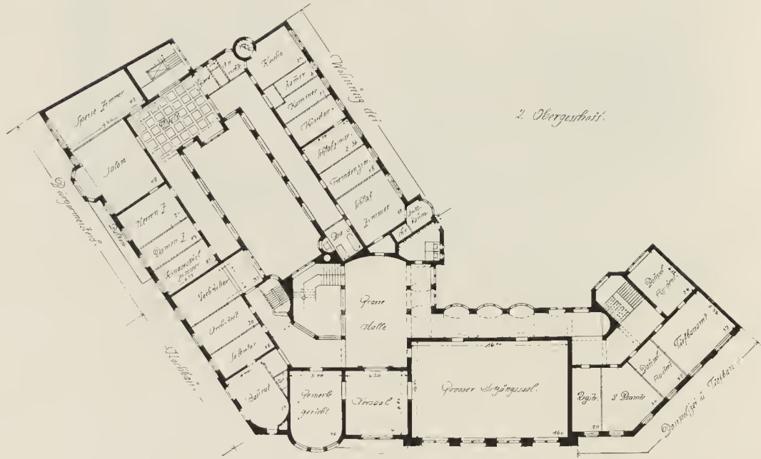
Josef Reuters-Wilmersdorf, Grundrisse zu dem Rathause für die Stadt Friedenau
