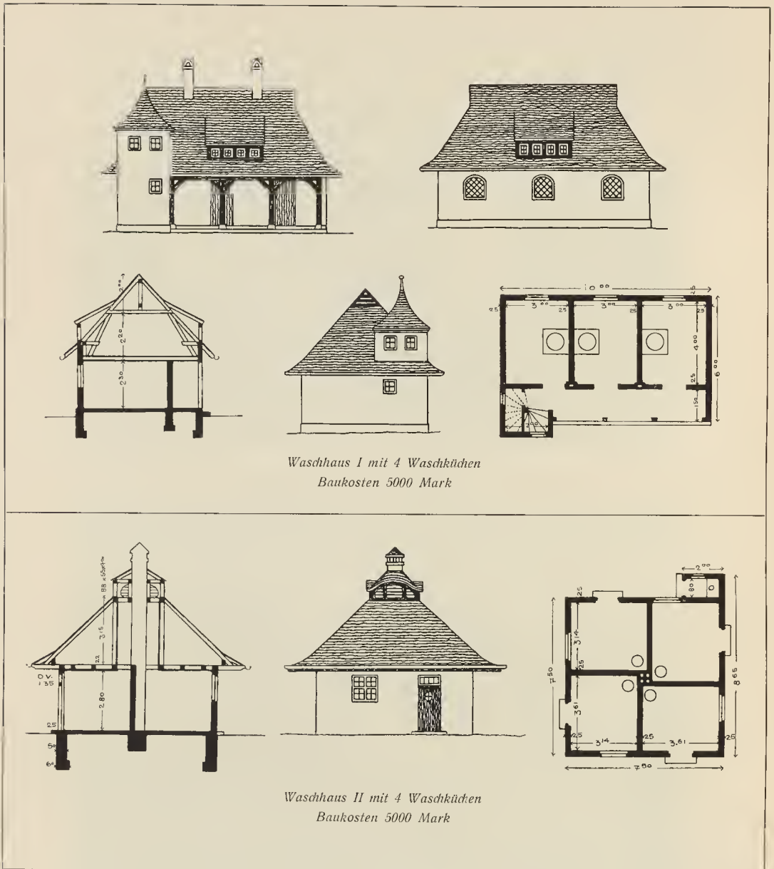
Arbeiterkolonie Gmindersdorf Waschhäuser
