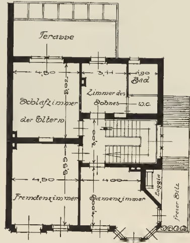
Grundrisse der Häuser Wolfes & Ehrlich in Breslau und Dr. Mäusch in Mors a. Rh.
