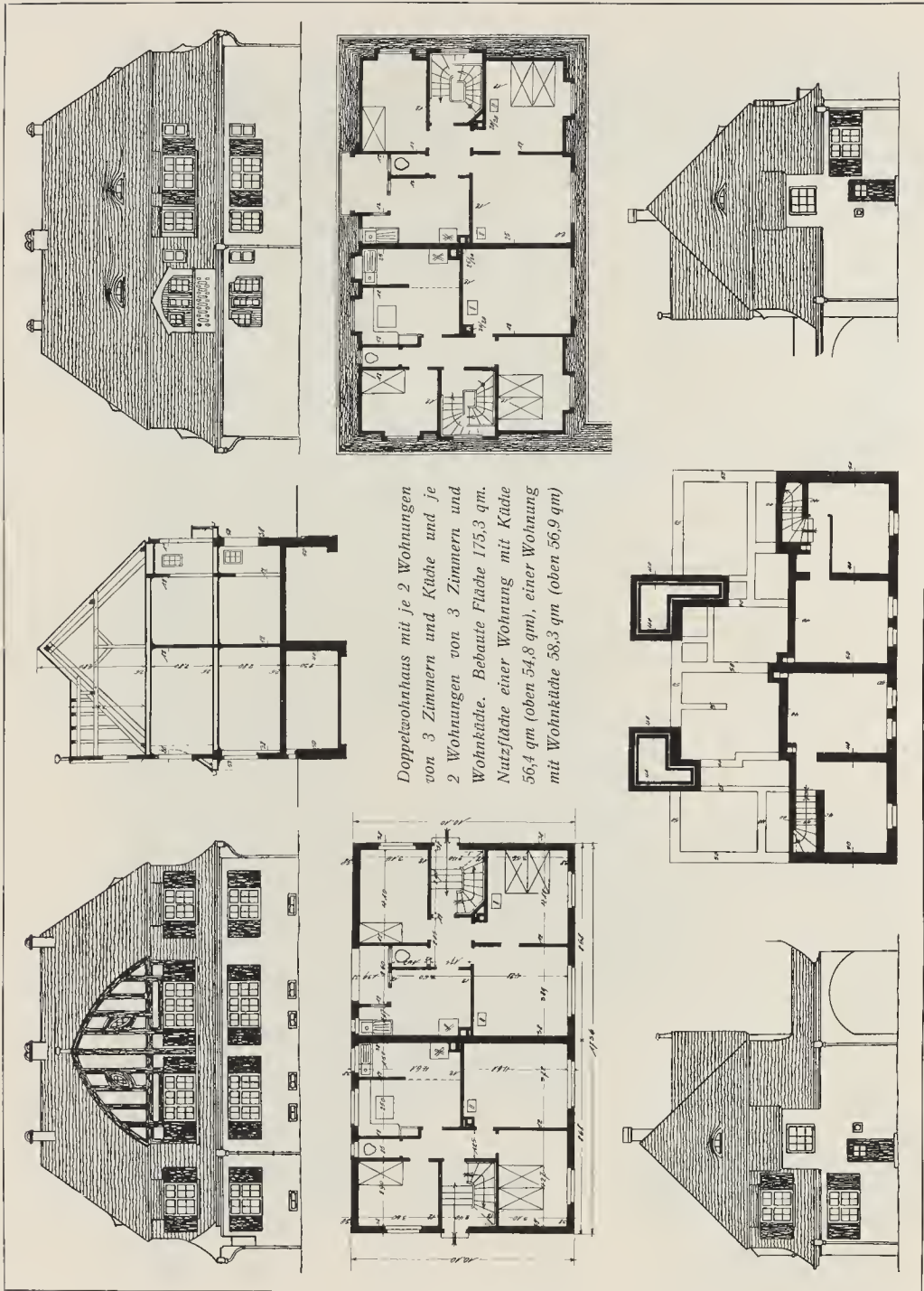
Arbeiterkolonie Gmindersdorf Haustype 15, Baukosten 21 000 Mark
