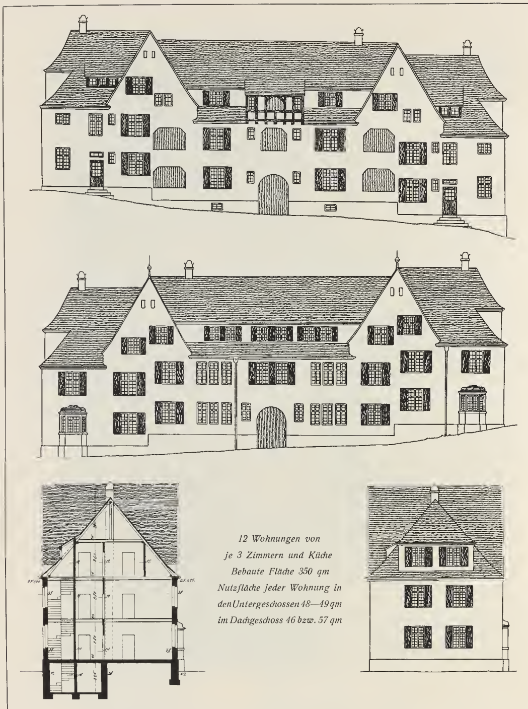
Arbeiterkolonie Gmindersdorf Reihenhaus, Baukosten 53000 Mark
