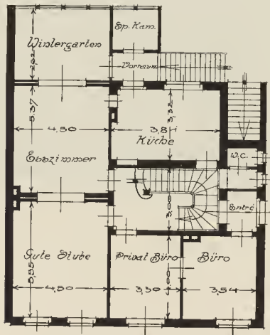
Grundrisse der Häuser Wolfes & Ehrlich in Breslau und Dr. Mäusch in Mors a. Rh.
