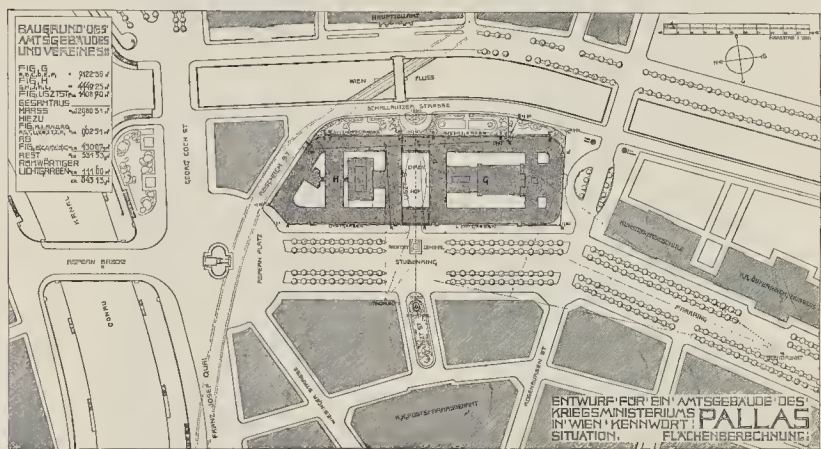
OBERBAURAT PROF. OTTO WAGNER-WIEN Grundrisse und Lageplan zum Wettbewerb für das Kriegsministerium in Wien
