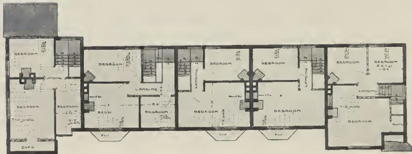
B. PARKER & R. UNWIN-YORK Haus für fünf Familien in Lettsworth
