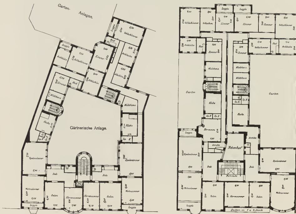
Grundrisse der Häuser Grolmanstrasse 3 und Bismarckstrasse 108
