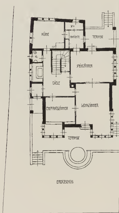
Hugo Eberhardt, Grundrisse der Häuser Wasels und Plappert
