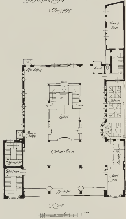
Kaufhaus M. Schneider in Neßtauben.
