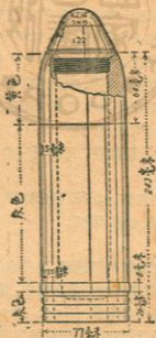
第六十六圖 1915 年式的 7.7 厘米綠十字砲彈
