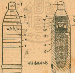
第七十九圖 十八磅砲芥氣砲彈
