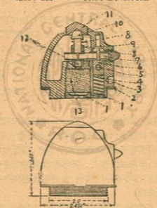
第四十七圖 M—XI 式化學迫擊砲彈引信
