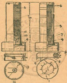
第四十八圖 司托克迫擊砲的發射藥
