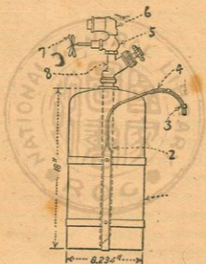
第三十九圖 輕便化學吹放瓶 M-I
