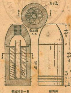
截面圖 B—B
