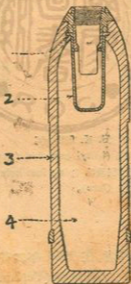
第六十五圖 75 毫米致命砲彈
