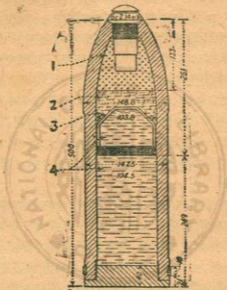
第七十六圖 15 厘米雙黃十字毒氣砲彈 (15-cm. double yellow cross gas shell)
