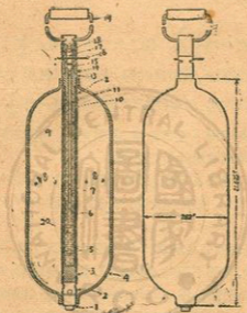
第四十一圖 李文氏投射砲砲彈，標號 II
