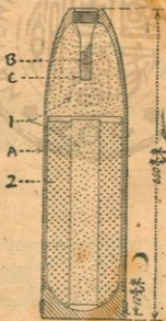
第八十三圖 17 厘米中型迫擊砲縱火彈
