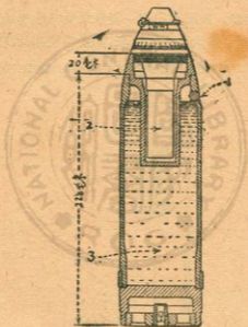
第七十圖 7.7 厘米迫擊砲毒氣彈（最後形式的 D 式迫擊砲彈）
