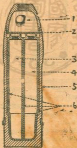
第六十二圖 75 毫米催淚砲彈
