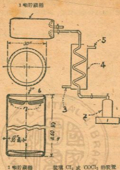
第五十一圖 戰場裝填站
