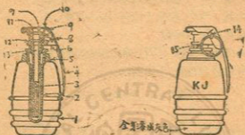
第二十九圖 美國第二號毒氣手榴彈
