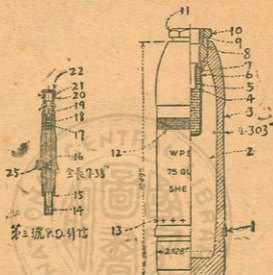
第二號 75 毫米砲彈 (黃磷彈的專用標記)
