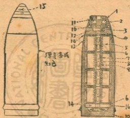
第八十六圖 4.5 英寸縱火榴彈砲彈
