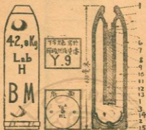
第五十九圖 17 厘米毒氣迫擊砲彈
