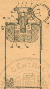
第三十四圖 第二號 H.C. 發煙燭
