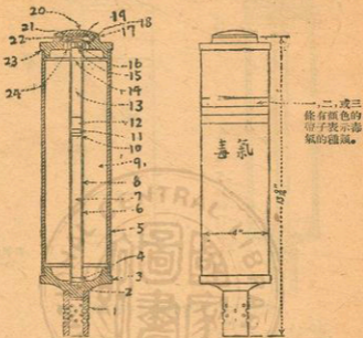
第四十四圖 四英寸可托克迫擊砲的毒氣彈
