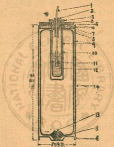
第五十八圖 9 厘米毒氣迫擊砲彈
