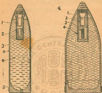
第七十一圖 17 厘米迫擊砲毒氣彈 (D式迫擊砲彈內裝光氣)
