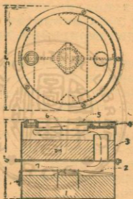
第五十圖 M-I 式 DM 刺激燭
