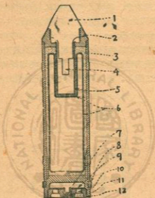
第六十一圖 輕型7.6厘米毒氣迫擊砲彈(即最初的C式砲彈)
