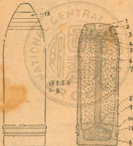
第八十五圖 十八磅砲縱火砲彈
