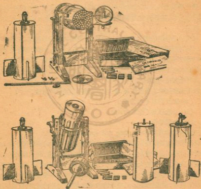
第九十八圖 英國罐形飛機縱火彈
