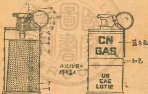
第三十圖 第七號催淚手榴彈
