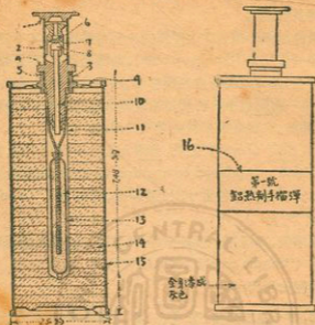
第三十一圖 第一號鋁熱劑手榴彈
