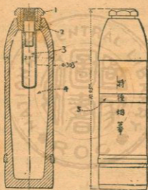
第八十圖 美國 75 毫米化學砲彈
