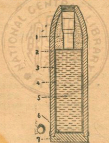
第五十六圖 十五厘米重野戰榴彈砲的 T-砲彈
