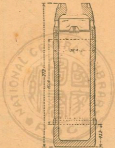
第八十七圖 美國 75 毫米縱火砲彈 [探準彈 (tracer shell)]
