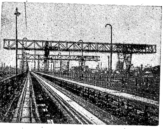
鞍鋼正在興建4座新式的煉焦爐。這項工程在今年3月動工，預計明年11月可以竣工。這項工程建成後，產量比現有鋼廠的7座煉焦爐生產的焦炭還要多。這些焦炭除滿足鞍鋼現有鋼廠的需要外，還能供應其他工廠需要。煉焦爐機械化時煤場上已安裝好兩台巨大的翻斗車，它担负着將煤場全部時煤的搬運任務。(新華社記者楊龍門攝)
