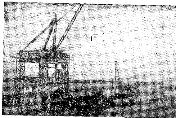
武漢鋼鐵聯合企業供水系統的 江心水塔站已開始興建，現在 正在長江的洪流中進行基礎工 程。這個水塔站基礎——鋼 圓筒比長江大橋最大的鋼筒還 要大三分之一。這是巨大的吊 機在江心水塔站基礎上打下了第 一根管樁。
