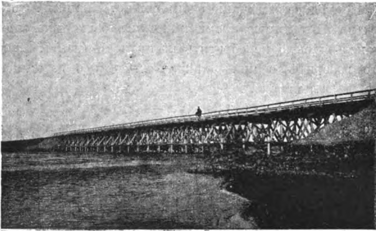
Мостъ Самаркандо-Андижанской желѣзвой дороги черезъ Заровшанъ.
