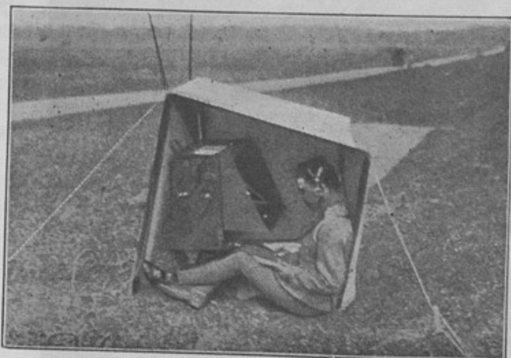
Безпроводный телеграфъ въ англійской арміи на полѣ сраженія. Приемъ депешъ.
